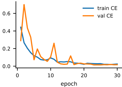
Classifier: cross-entropy
