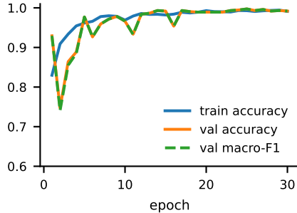
Classifier: accuracy / macro-F1
