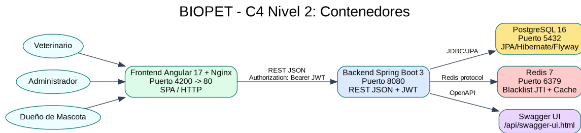
Figure 1: Diagrama C4 Nivel 2 (contenedores) de BIOPET, generado a partir de la configuración real de docker-compose.yml .
