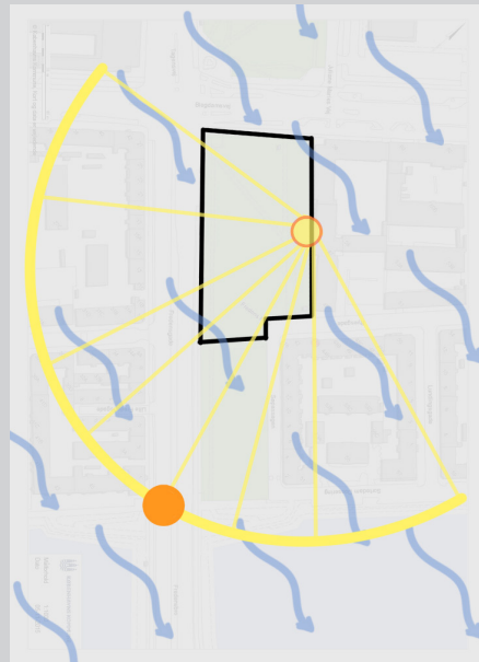
Sun
