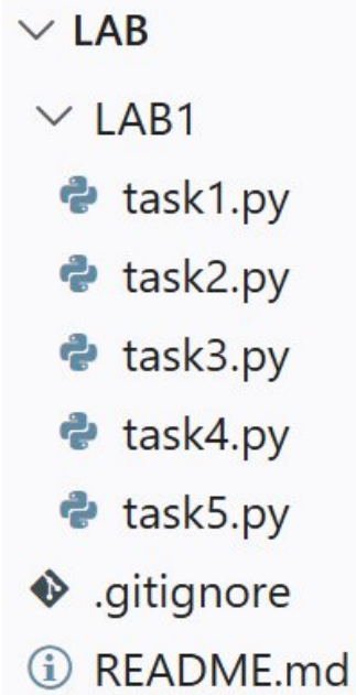
Рисунок 2 – Структура репозитория
