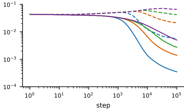
MSE
