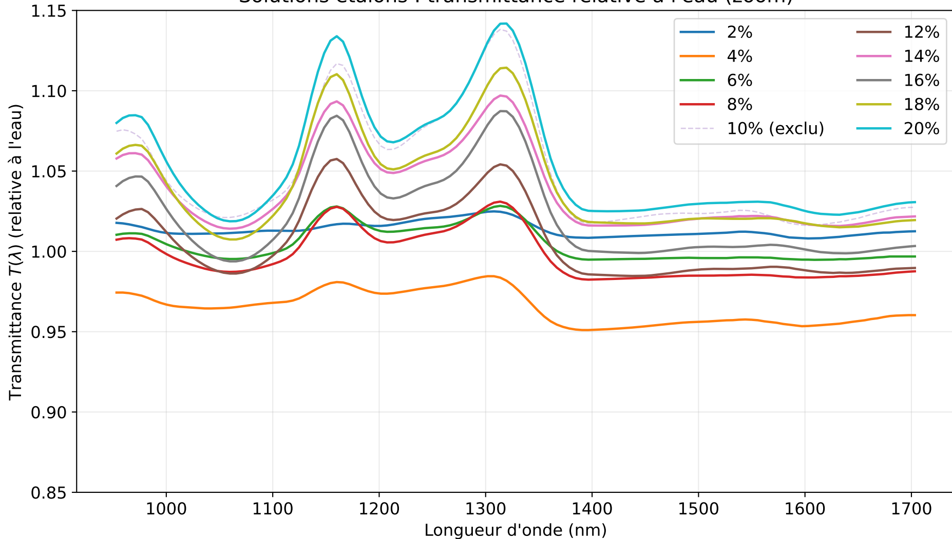
Solutions étalons : transmittance relative à l'eau (zoom)
