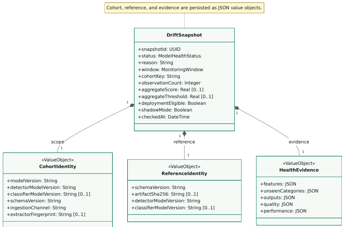
Figure 3.3 – Classes associées au suivi de l’état des modèles
