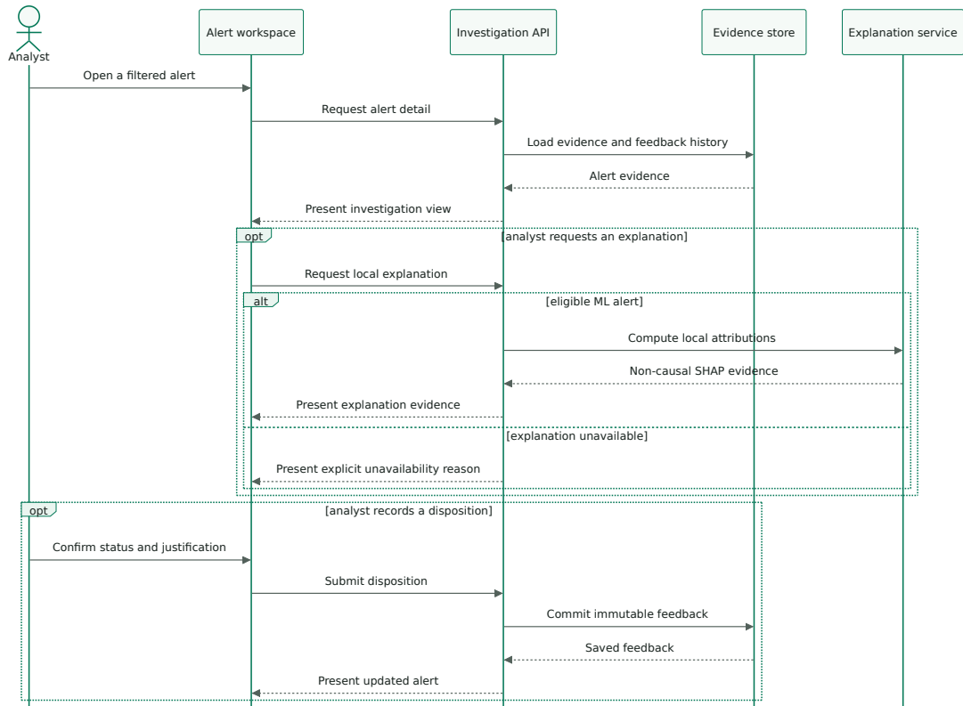
Figure 3.13 – Séquence d'investigation et de qualification d'une alerte
