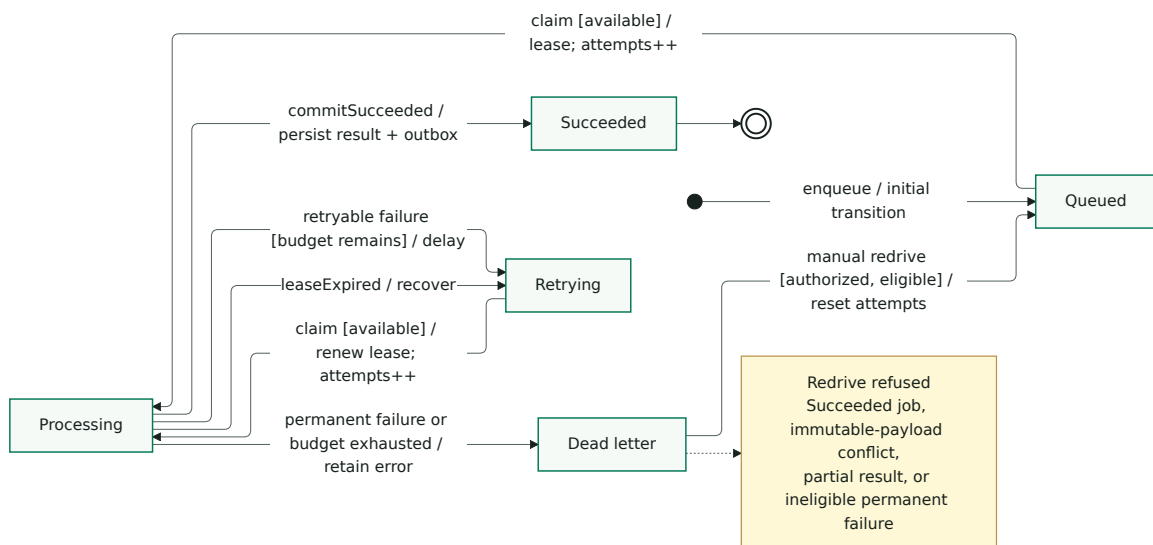
Figure 3.11 – Machine à états d’un travail d’ingestion
