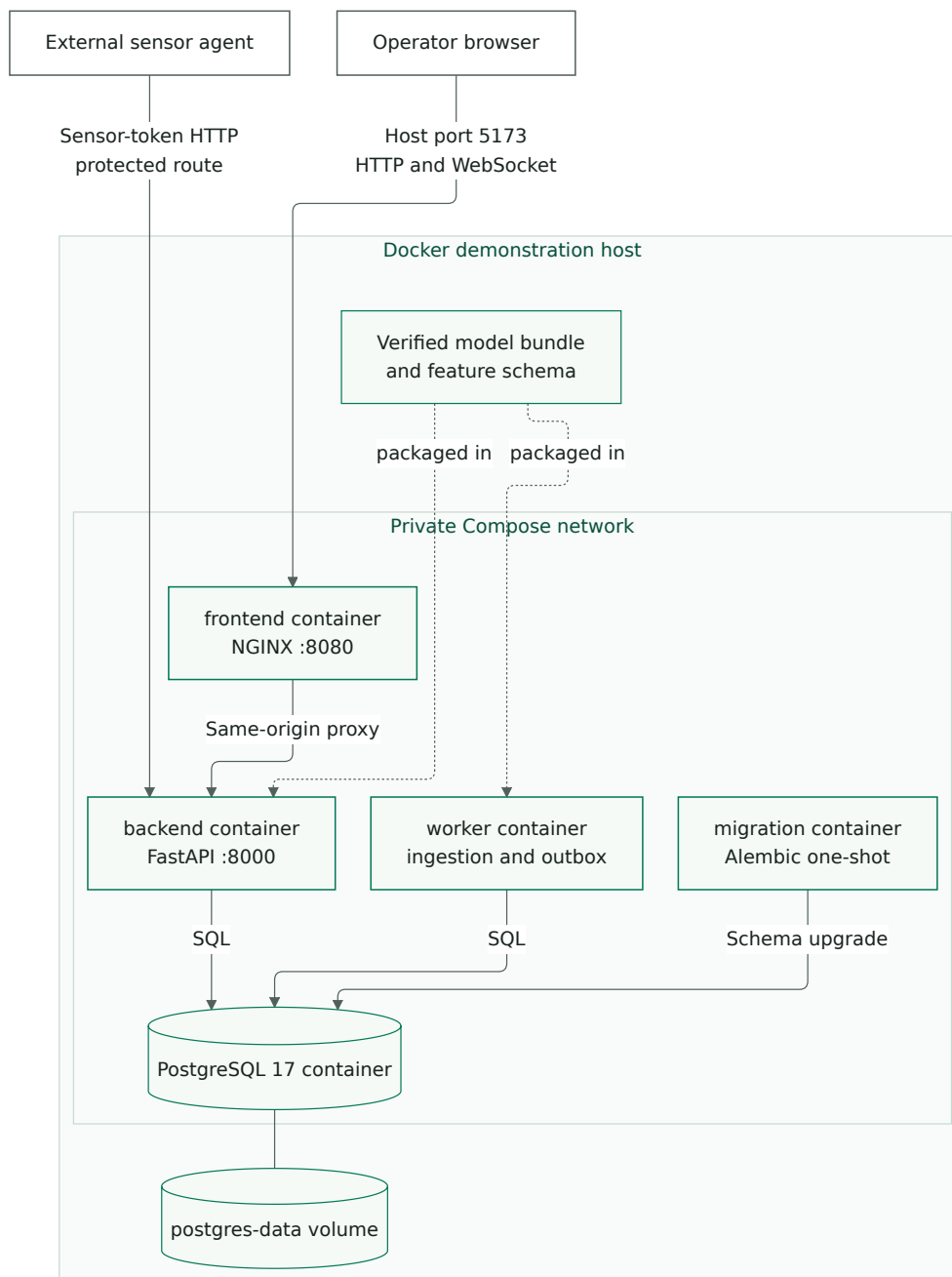
Figure 3.7 – Déploiement du mode de démonstration Docker
