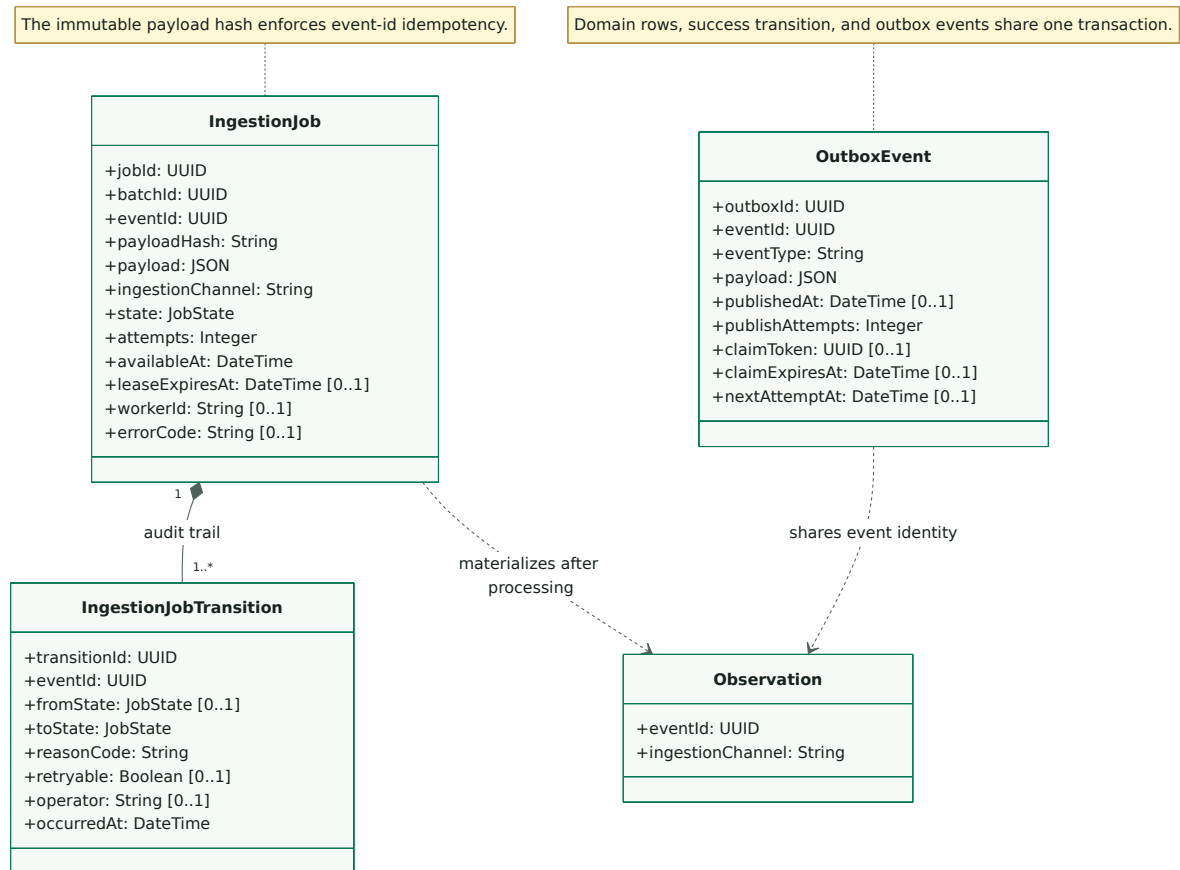
Figure 3.2 – Classes associées à l’ingestion durable
