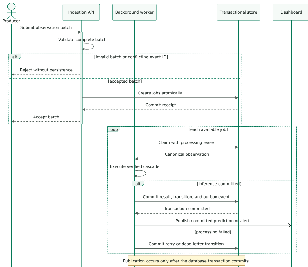
Figure 3.10 – Séquence d’ingestion durable et de diffusion des résultats
