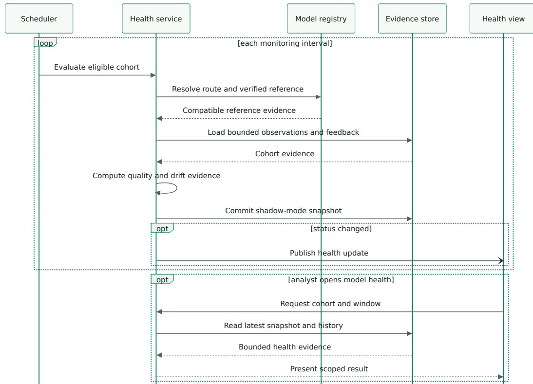
Figure 3.14 – Séquence de consultation de la santé d'un modèle
