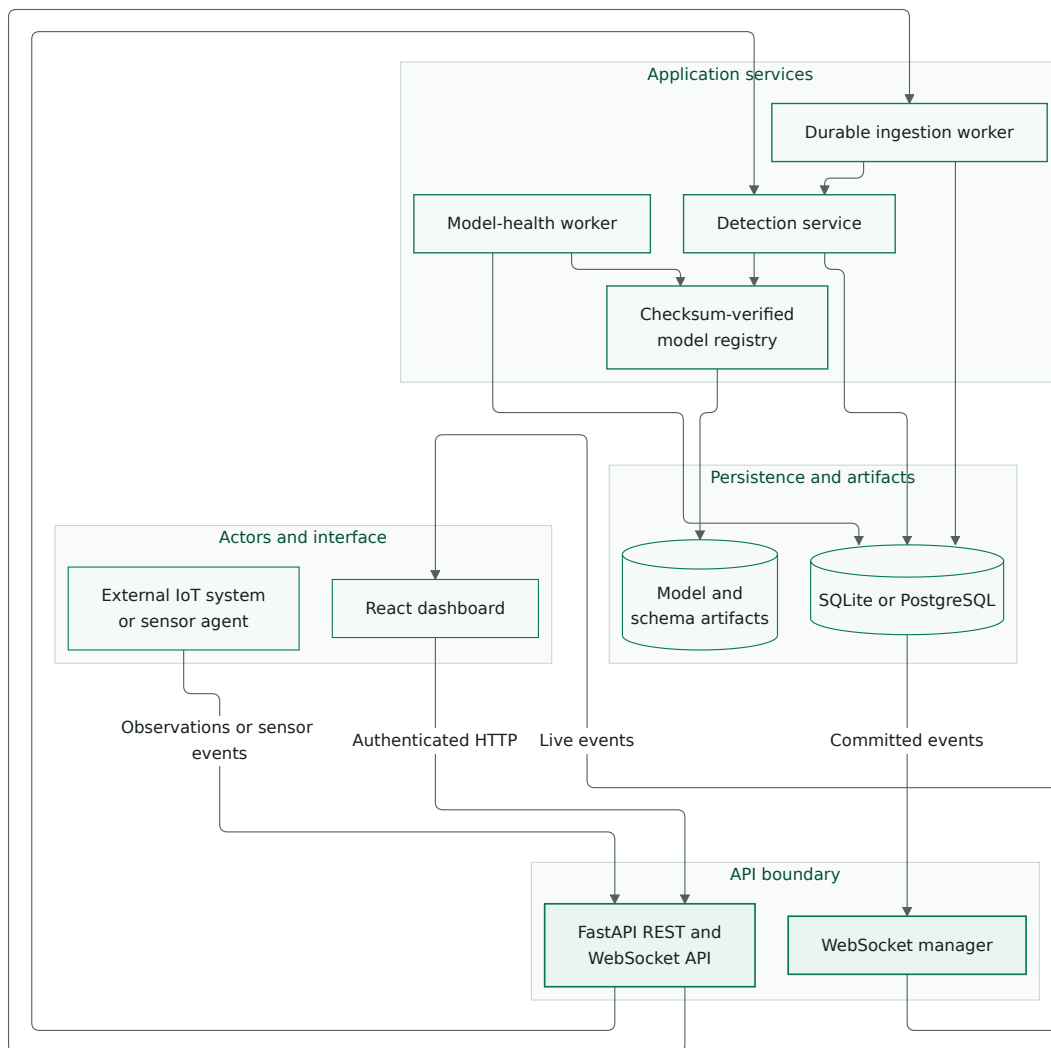
Figure 3.6 – Architecture logicielle par composants
