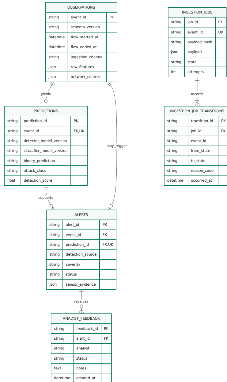
Figure 3.5 – Modèle relationnel du noyau de détection et d'ingestion
