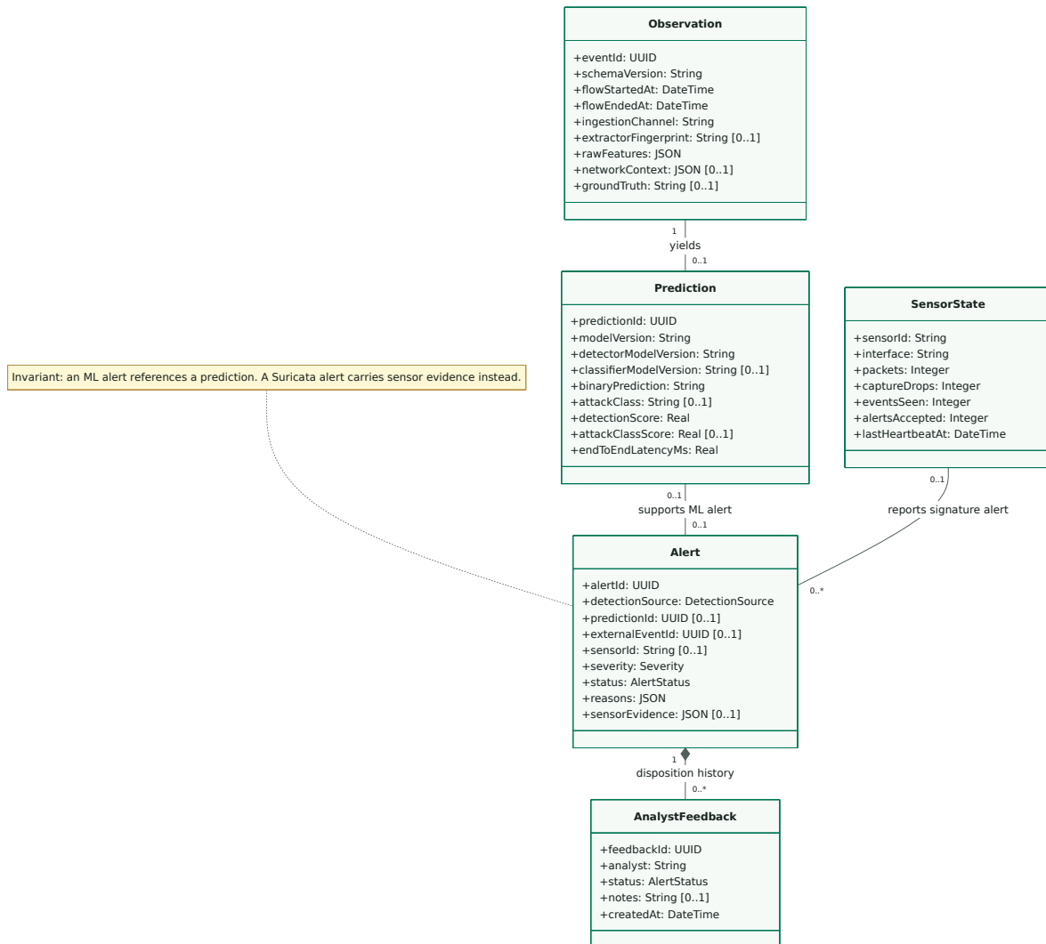
Figure 3.1 – Diagramme de classes du domaine principal
