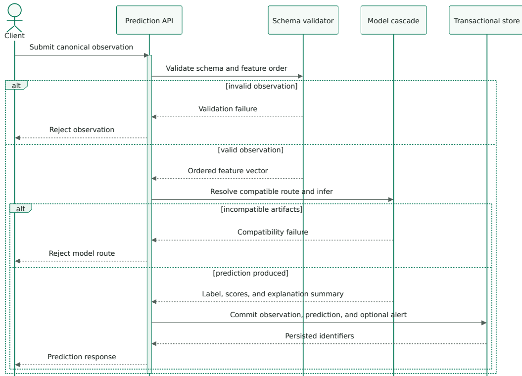
Figure 3.12 – Séquence de prédiction synchrone
