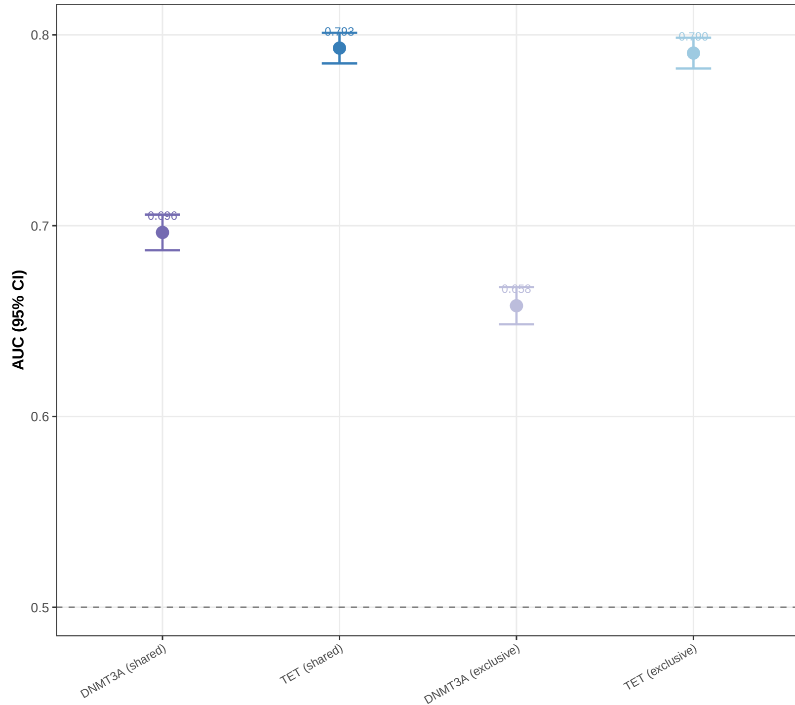
AUC Comparison
