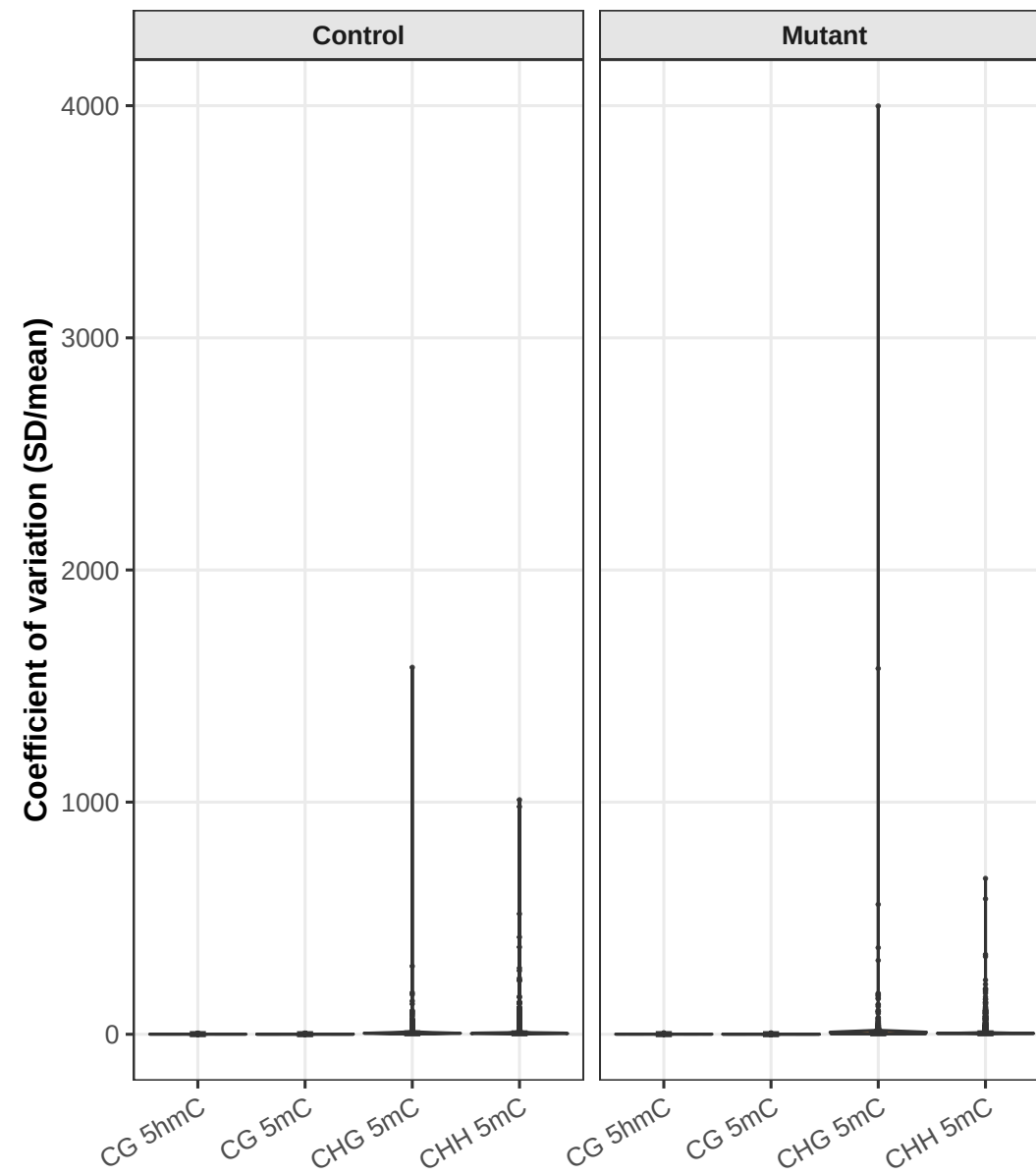
B. Intra-TAD CV
