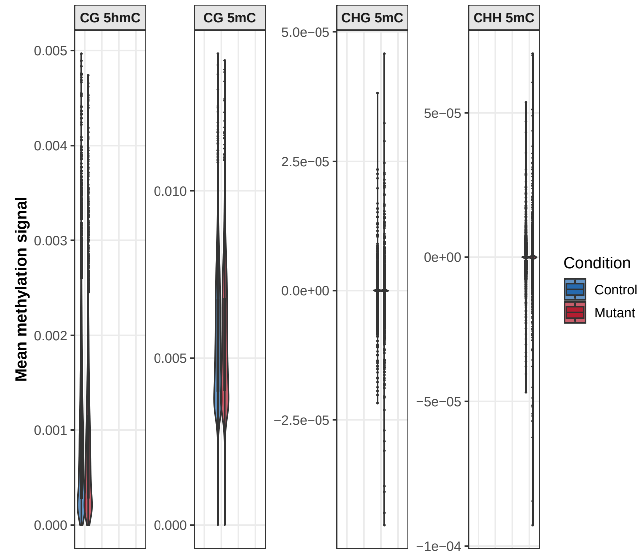
A. Signal per TAD
