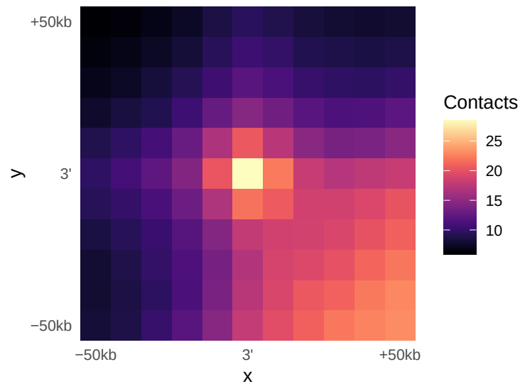
mut_M2
