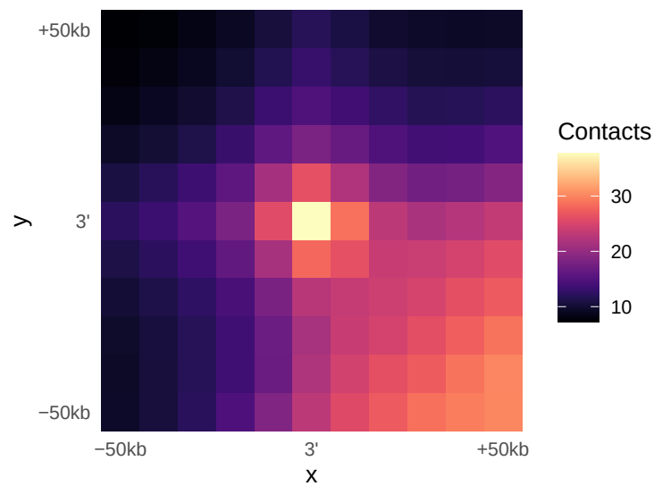
mut_M2
