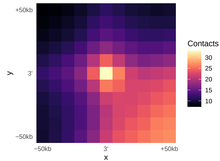
mut_M3
