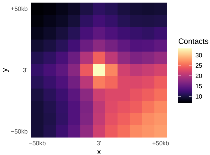
mut_M1
