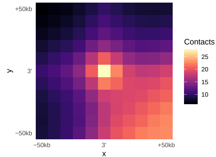
mut_M3
