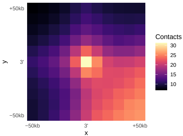
mut_M1
