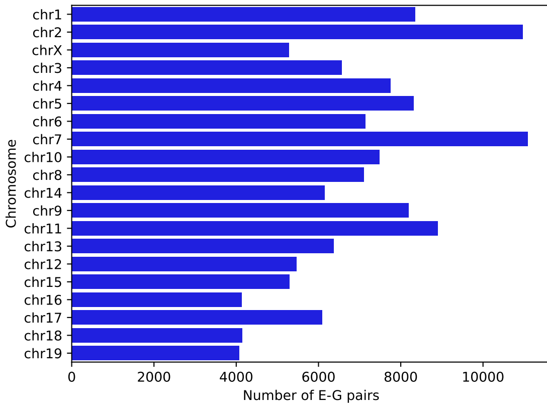
Enhancer-Gene Pairs Per Chromosome
