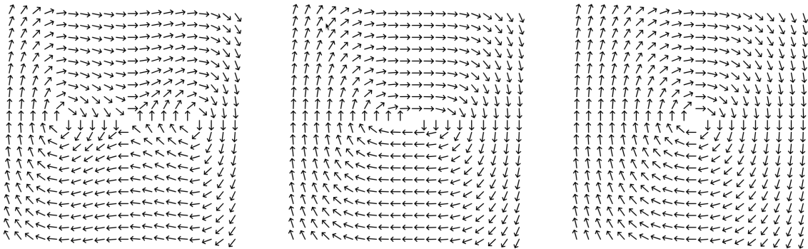
FIGURE 3 – Le champ de vecteur associé à 47 en \lambda = 0.85, 0 et -0.85
