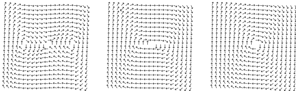
FIGURE 1 – Le champ de vecteur associé à 3 en \lambda = 0.85, 0 et -0.85
