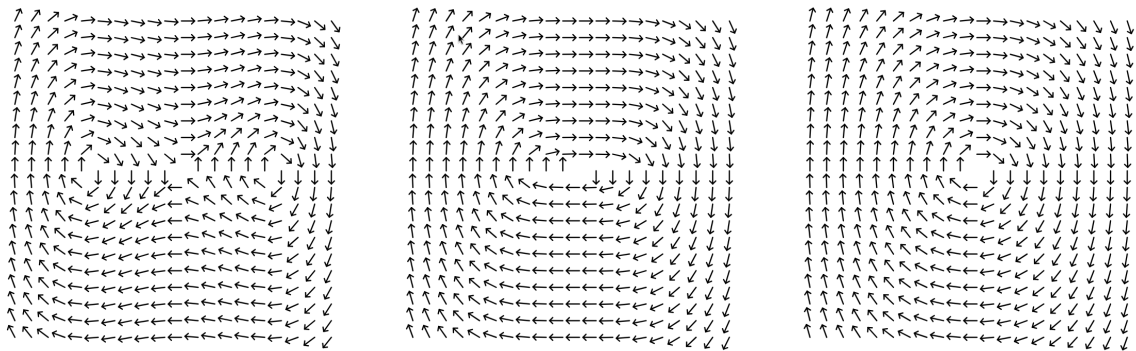
FIGURE 3 – Le champ de vecteur associé à 48 en \lambda = 0.85, 0 et -0.85
