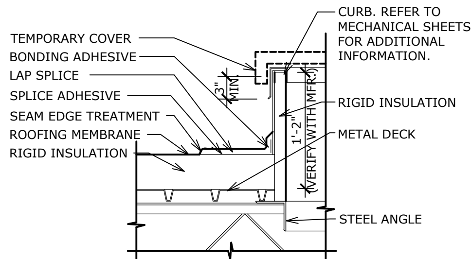
4 CURB DETAIL SCALE: 1" = 1'-0"
