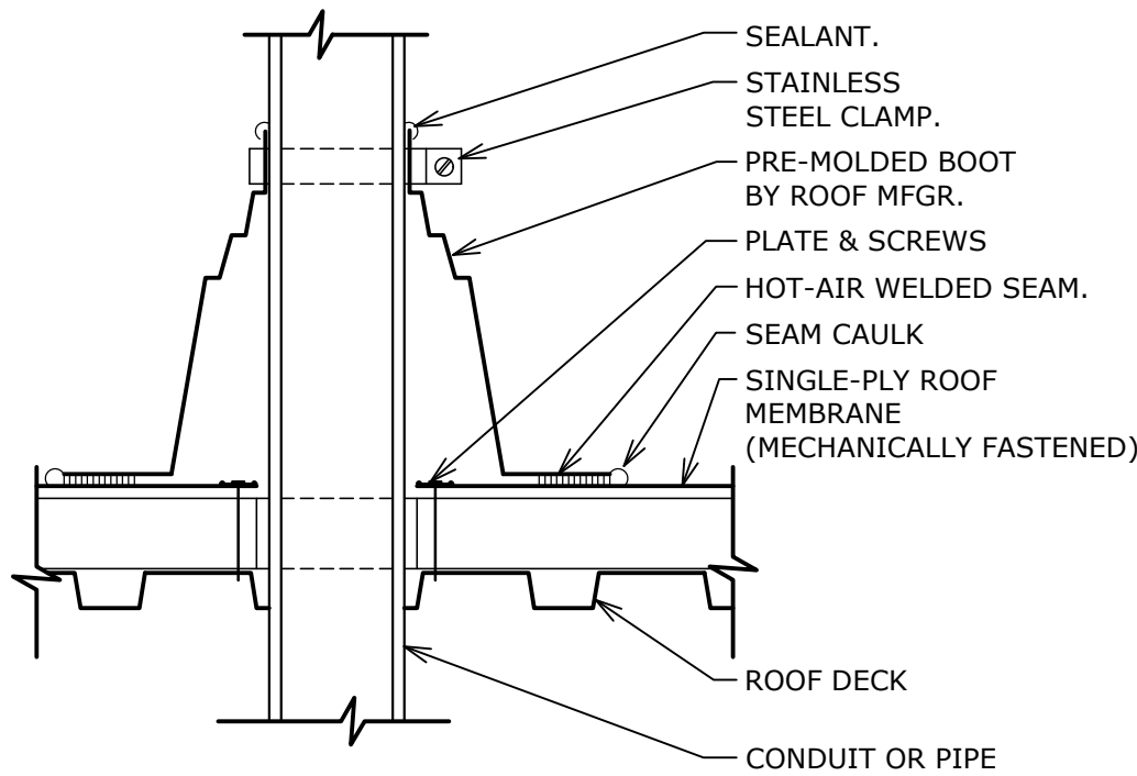
2 VENT PIPE DETAIL SCALE: 1" = 1'-0"
