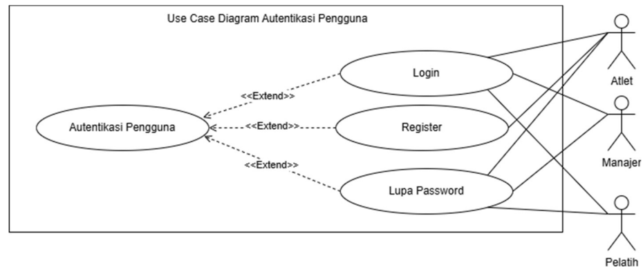
Gambar Use Case Diagram Autentikasi Pengguna
