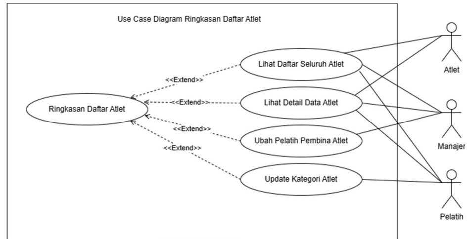
Gambar Use Case Diagram Lihat Ringkasan Daftar Atlet
