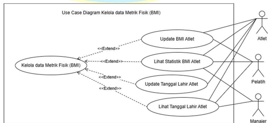
Gambar Use Case Diagram Kelola Data Metrik Fisik (BMI)
