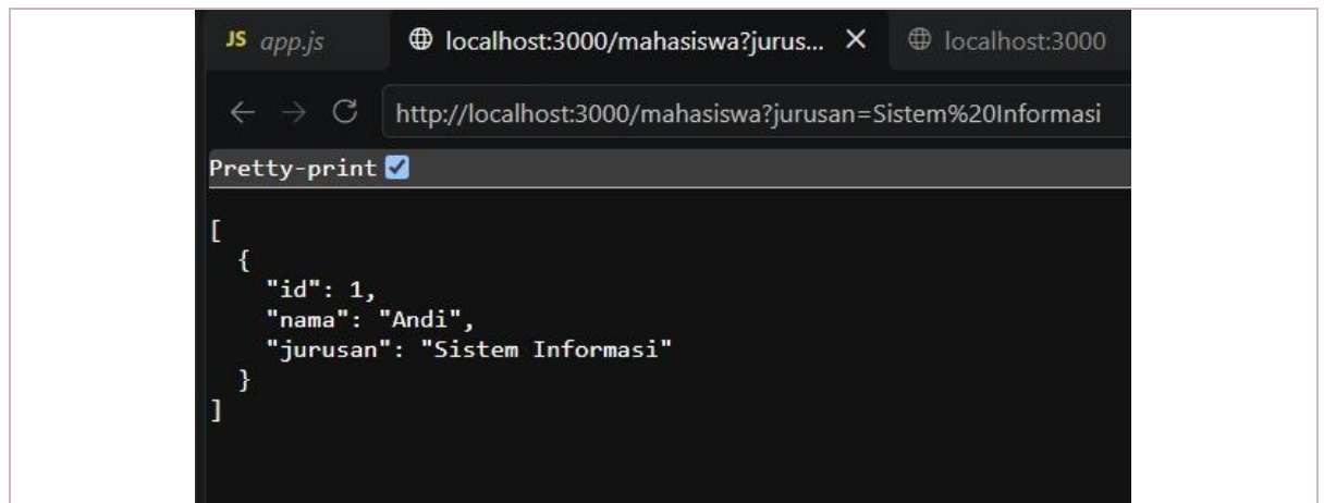
Gambar 5. Pengujian filter mahasiswa berdasarkan jurusan.
