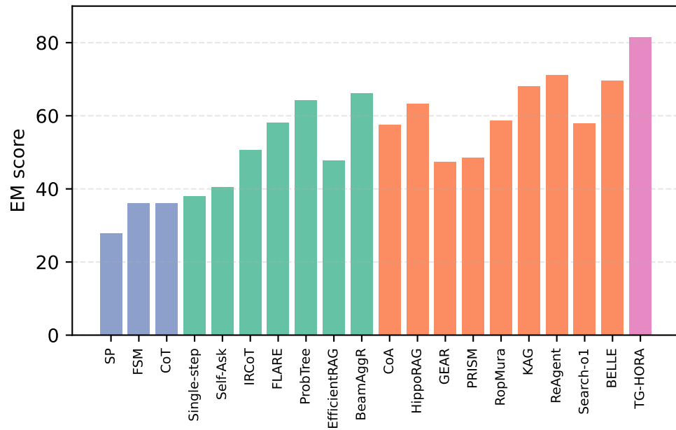
2WikiQA (EM)
