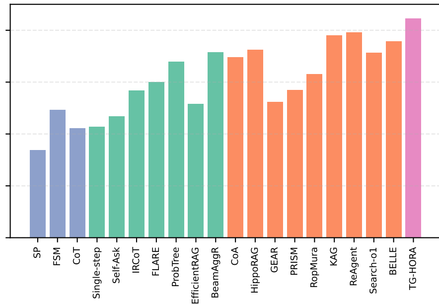
2WikiQA (F1)
