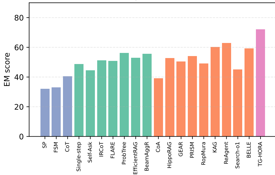
HotpotQA (EM)
