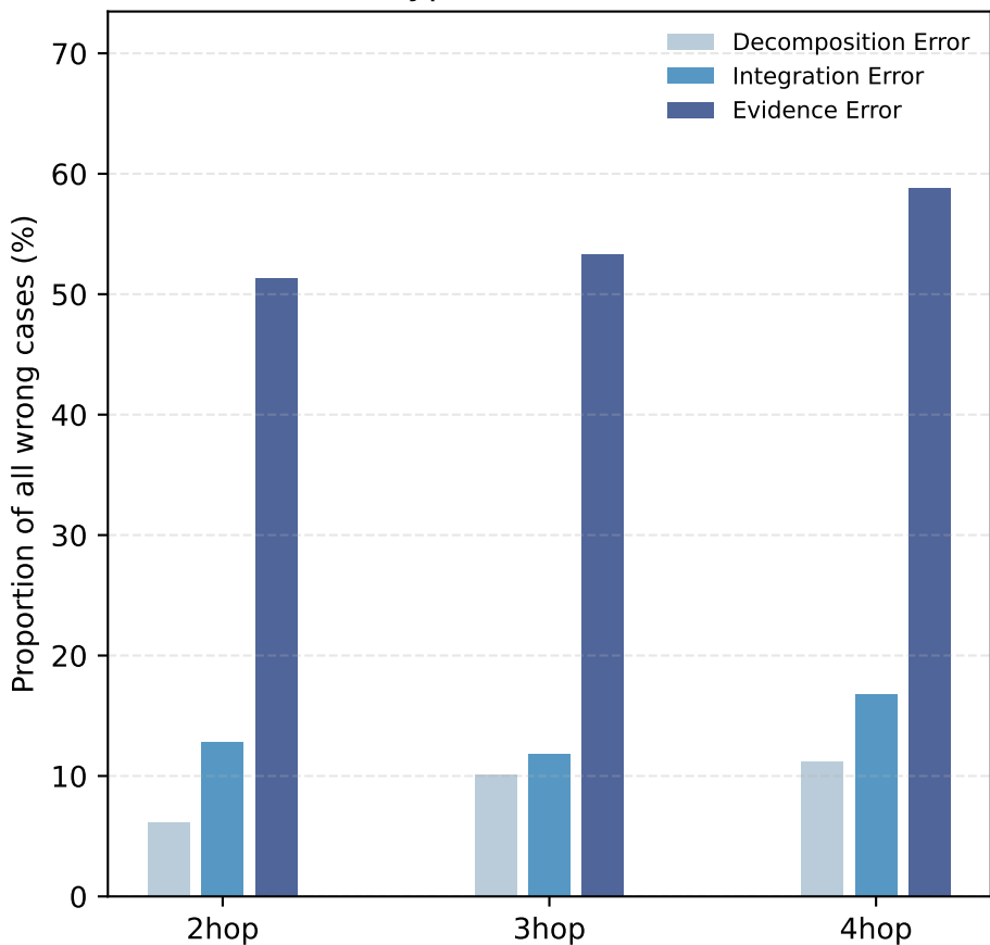
Error type ratios on MuSiQue
