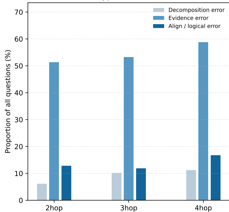
(a) Error type ratios on MuSiQue
