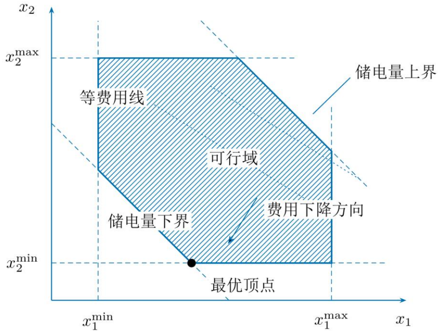
图 7 相邻两段可行域示意
