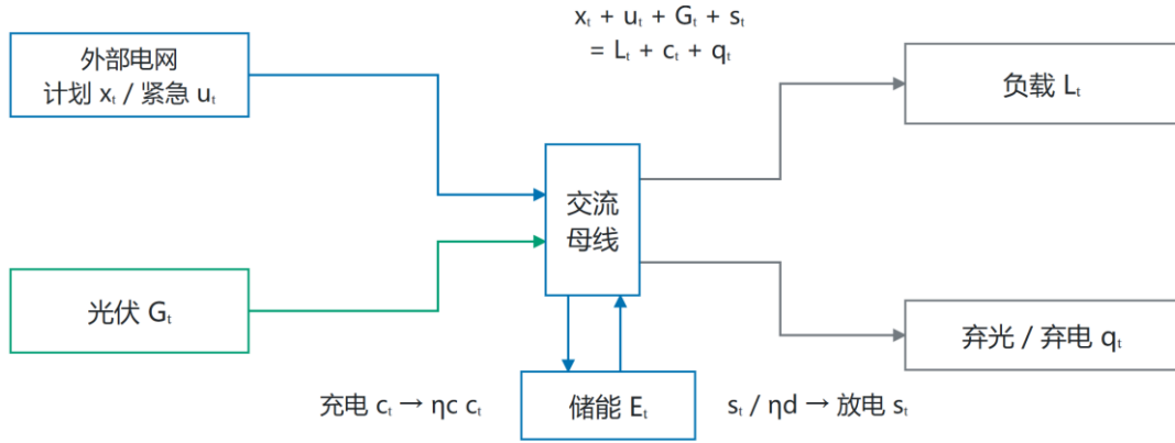
图 2 母线能量流与储能效率
