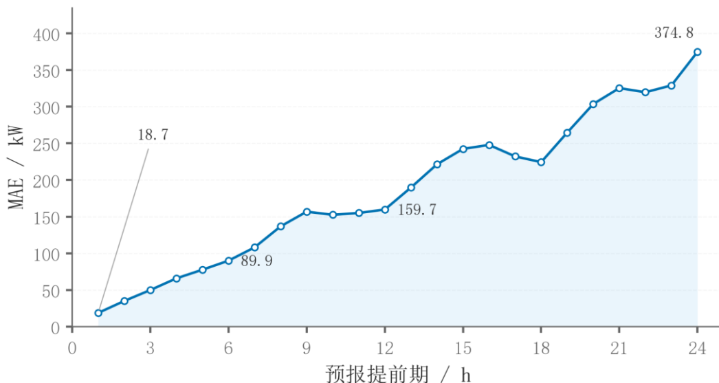
图 24 光伏预报误差随提前期变化
