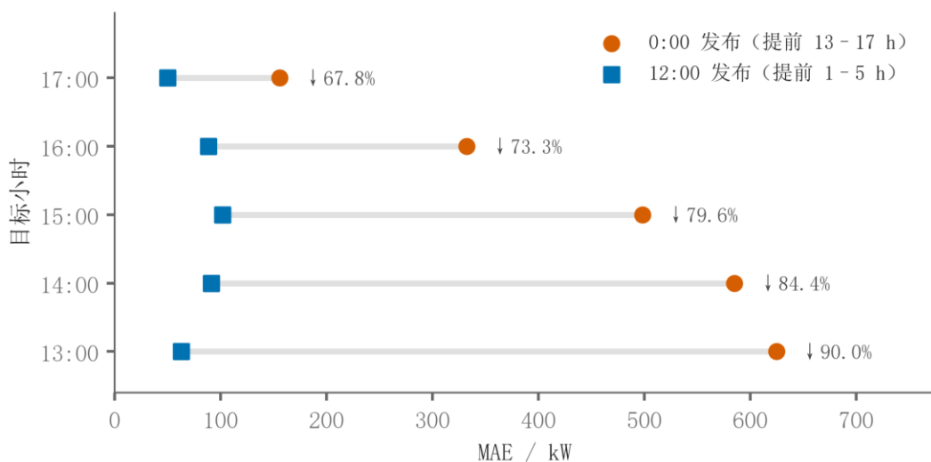
图 16 同目标不同发布时刻预报
