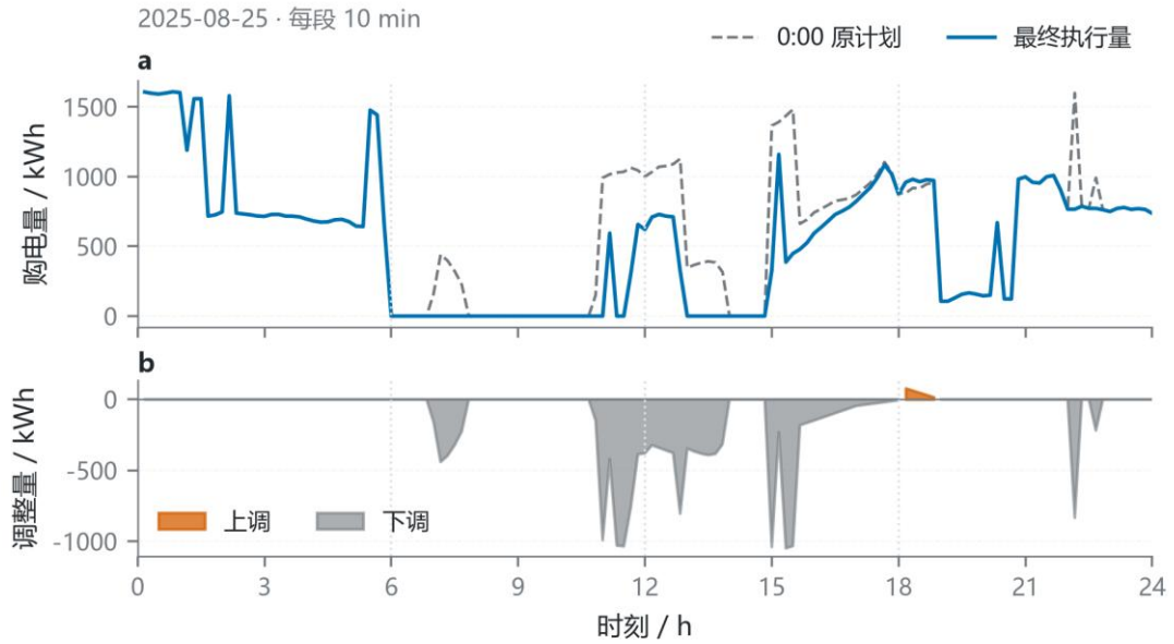
图 17 日前计划与滚动执行对照
