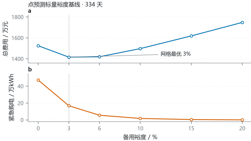
图 14 点预测基线的裕度与风险权衡
