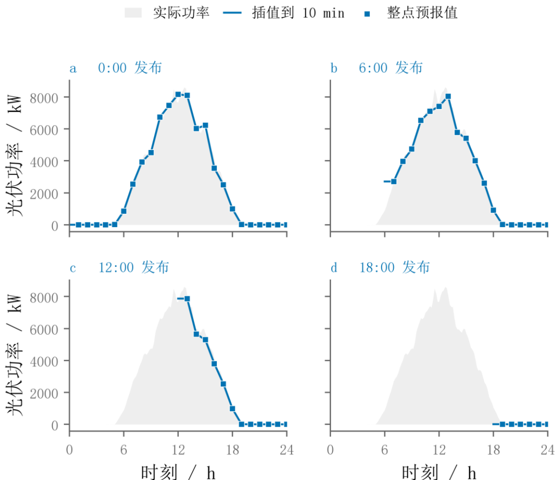
图 20 预报插值一致性核查
