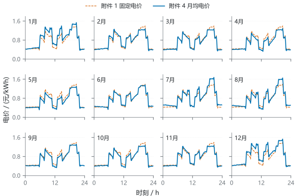
图 21 逐月电价与固定基准对照
