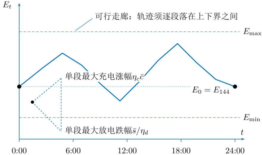
图 8 储电量可行走廊示意
