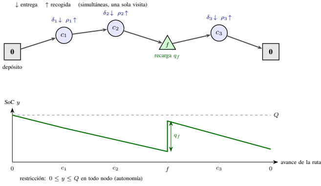
Fig. 1: Esquema del VRPSPDTW-E. Arriba: una ruta entrega (↓) y recoge (↑) en cada cliente y se desvía a una estación f para recargar q_f . Abajo: el estado de carga (SoC) decae con la distancia y se repone parcialmente en f , sujeto a 0 \leq y \leq Q .
