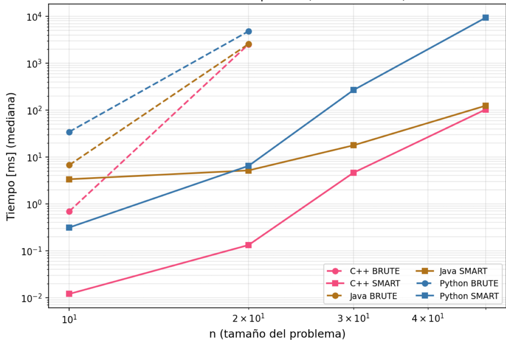
Escalabilidad: tiempo vs n (familia random)
