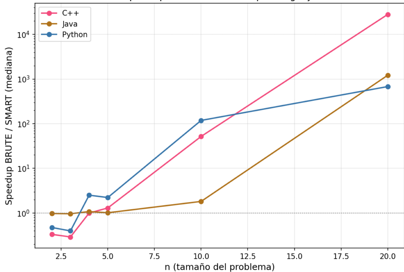
Speedup: BRUTE vs SMART por lenguaje
