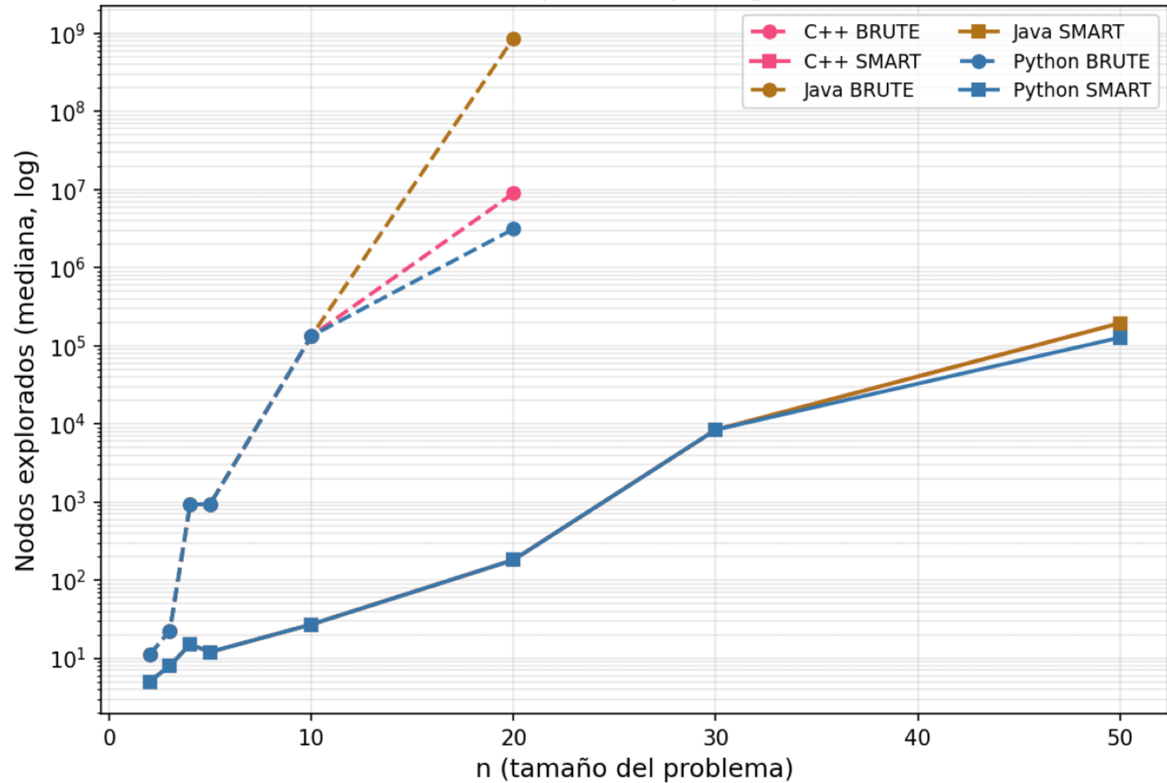
Nodos explorados por algoritmo
