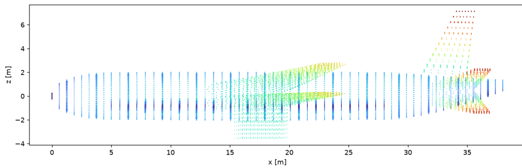
Mode 4, 0.89 Hz
