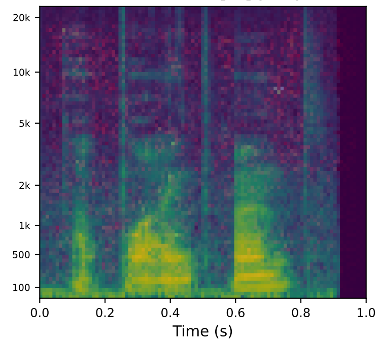
BROWSER [C5] (98%)
