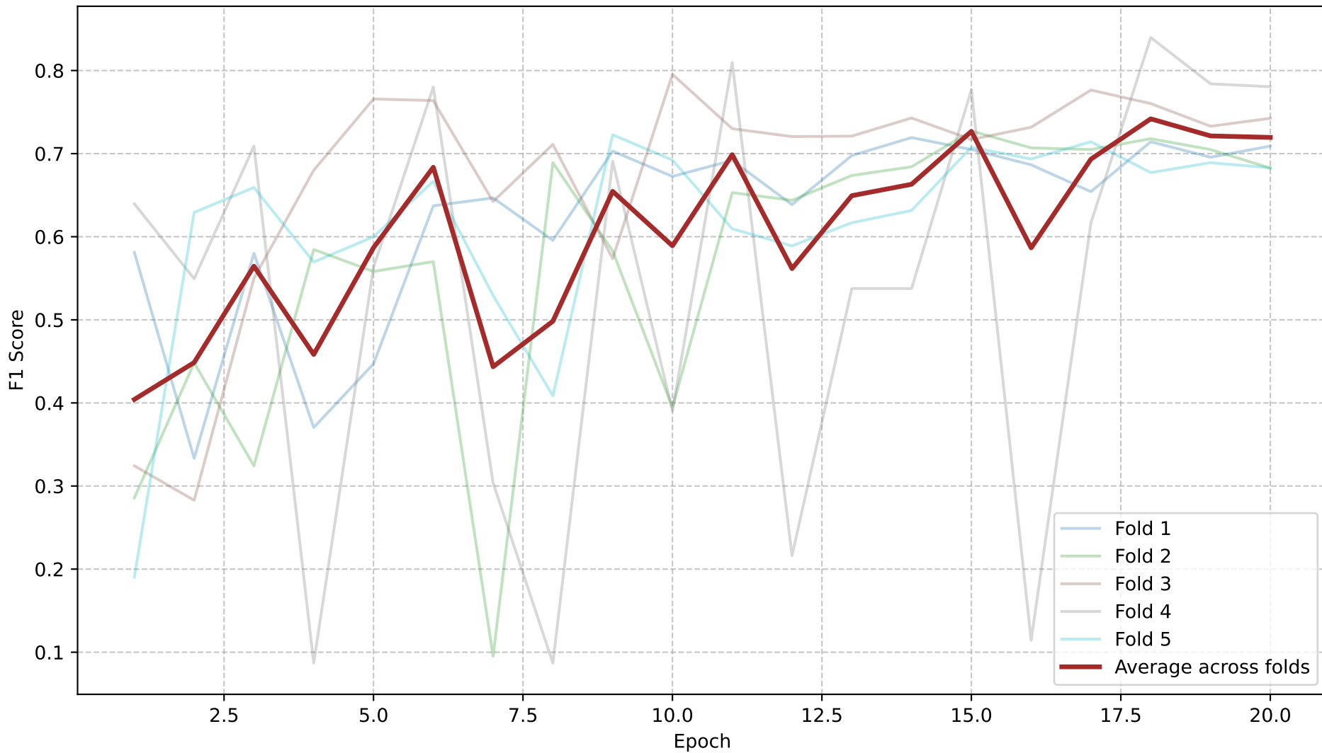
Validation F1 Score by Epoch
