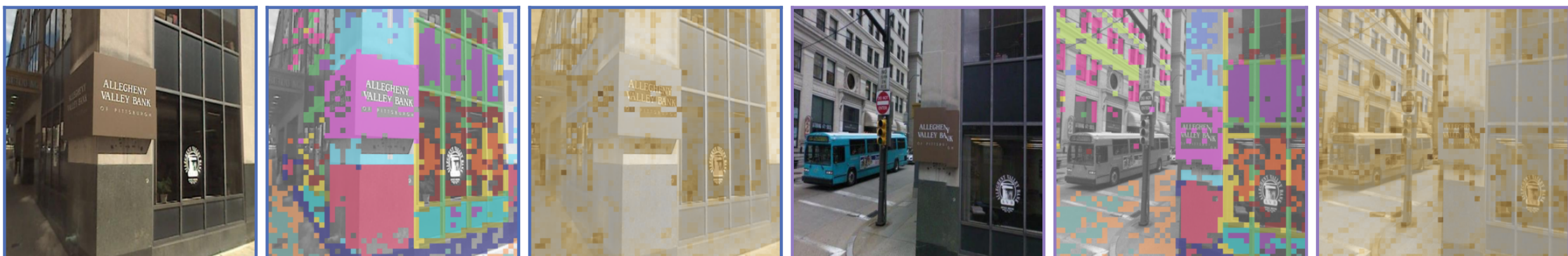
Pitts250k
