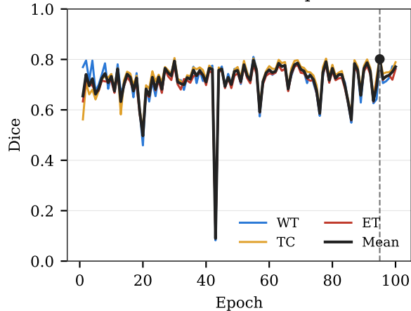
Validation Dice, best epoch 95
