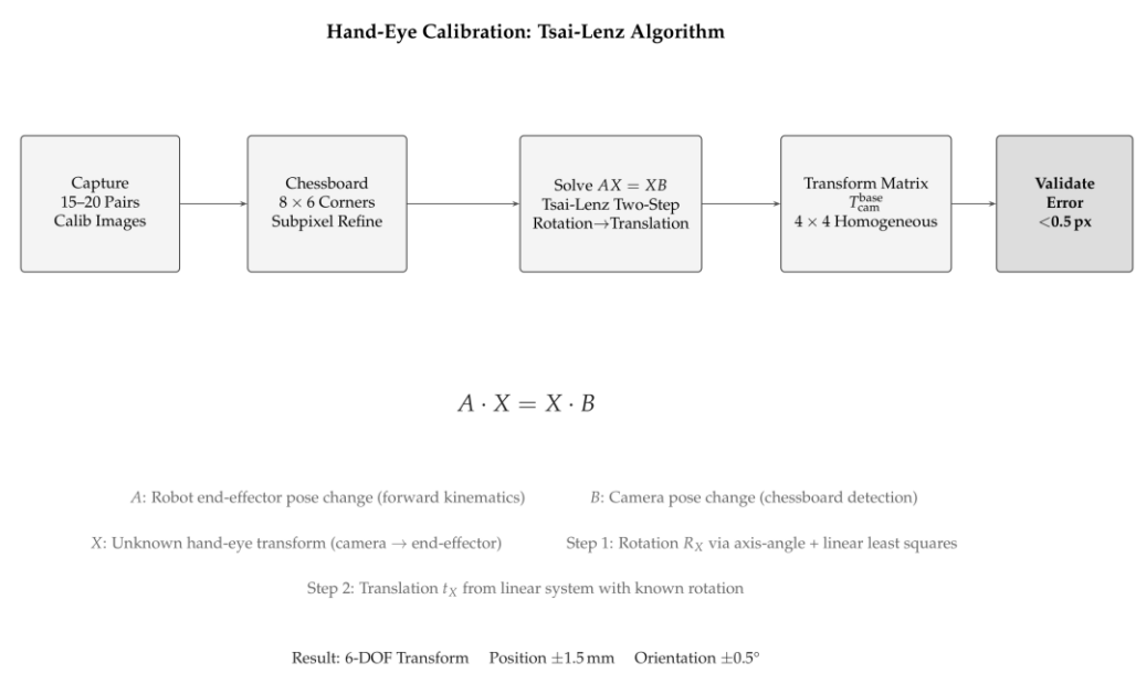
图 4-3 手眼标定流程（Tsai-Lenz 算法 AX=XB 求解）
