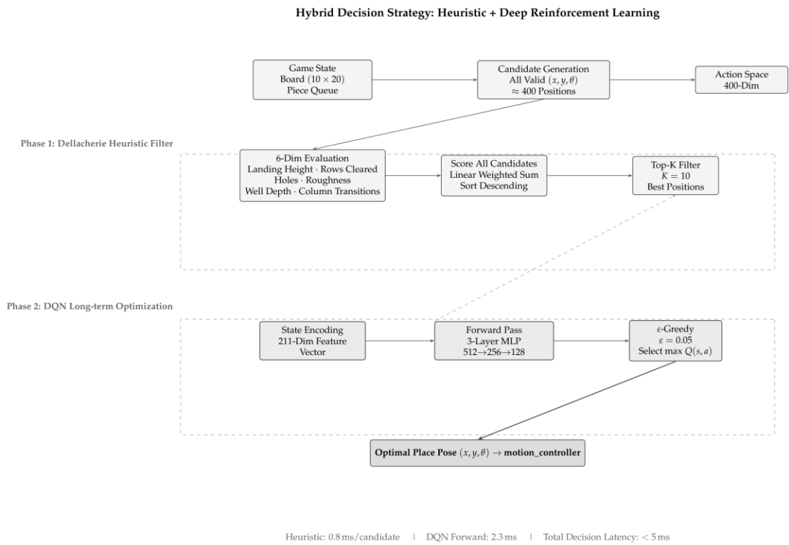
图 4-5 混合决策策略流程（Dellacherie 启发式筛选 + DQN 长期价值优化）
