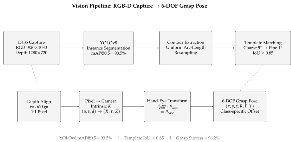
图 4-8 视觉识别流水线（D435 采集$ ightarrow$YOLOv8 分割$ ightarrow$模板匹配$ ightarrow$6-DOF 位姿）
