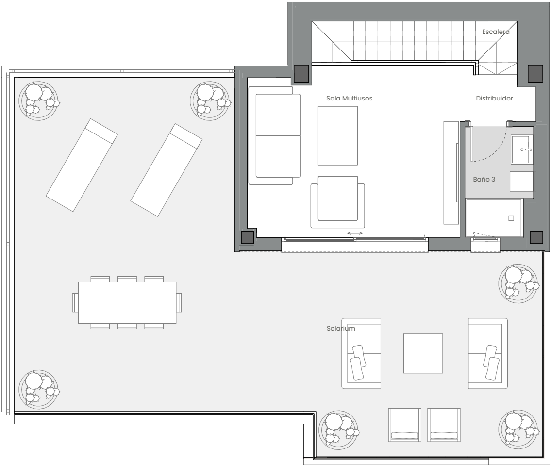
PLANTA SUPERIOR_P05
