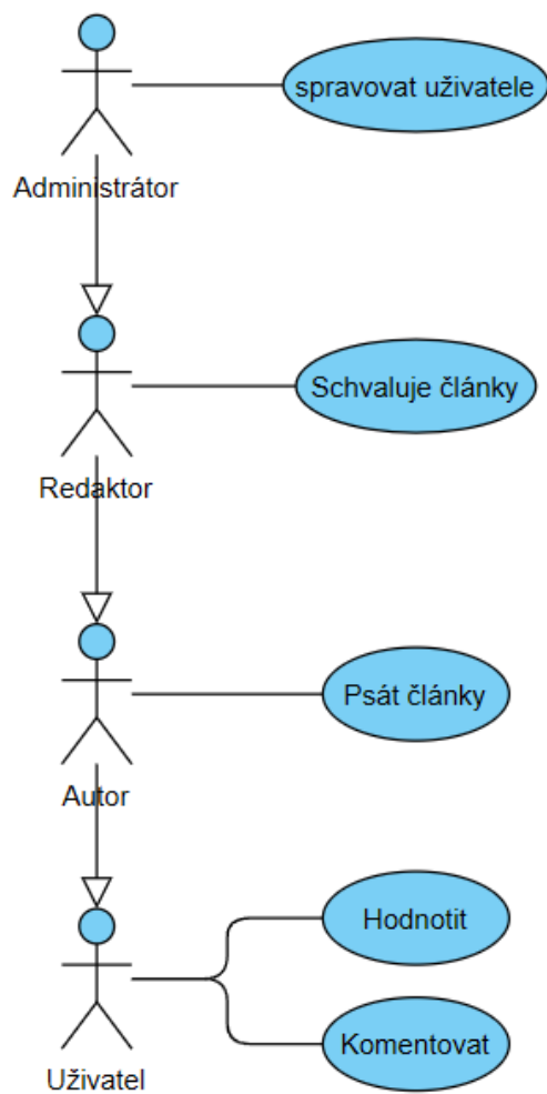
Obrázek 4 Use-Case diagram
