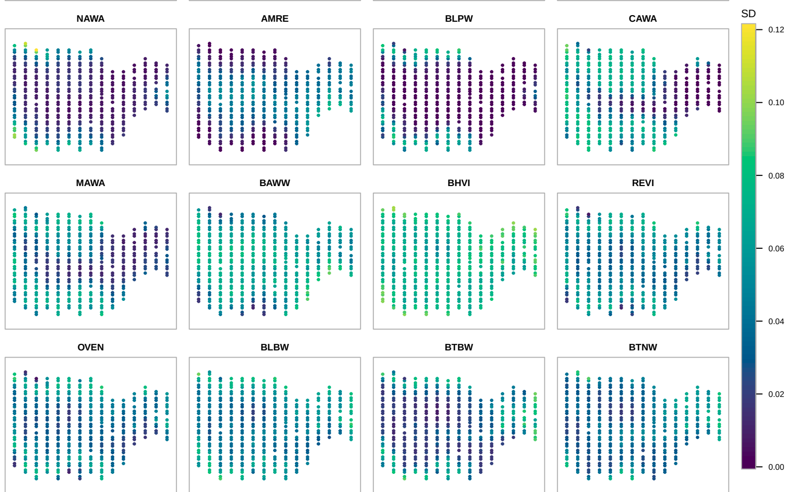
(b) posterior standard deviation
