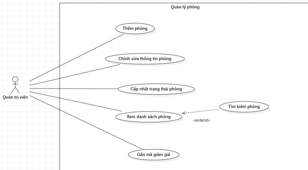
Use case Quản lý phòng
