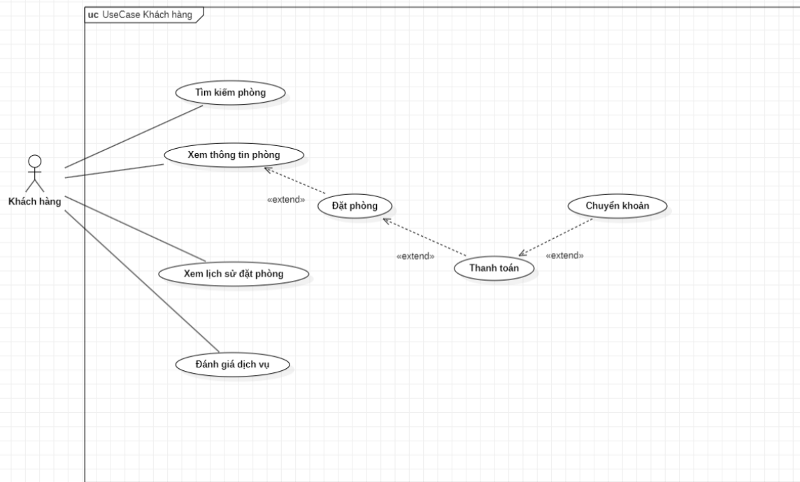
Use case Khách Hàng
