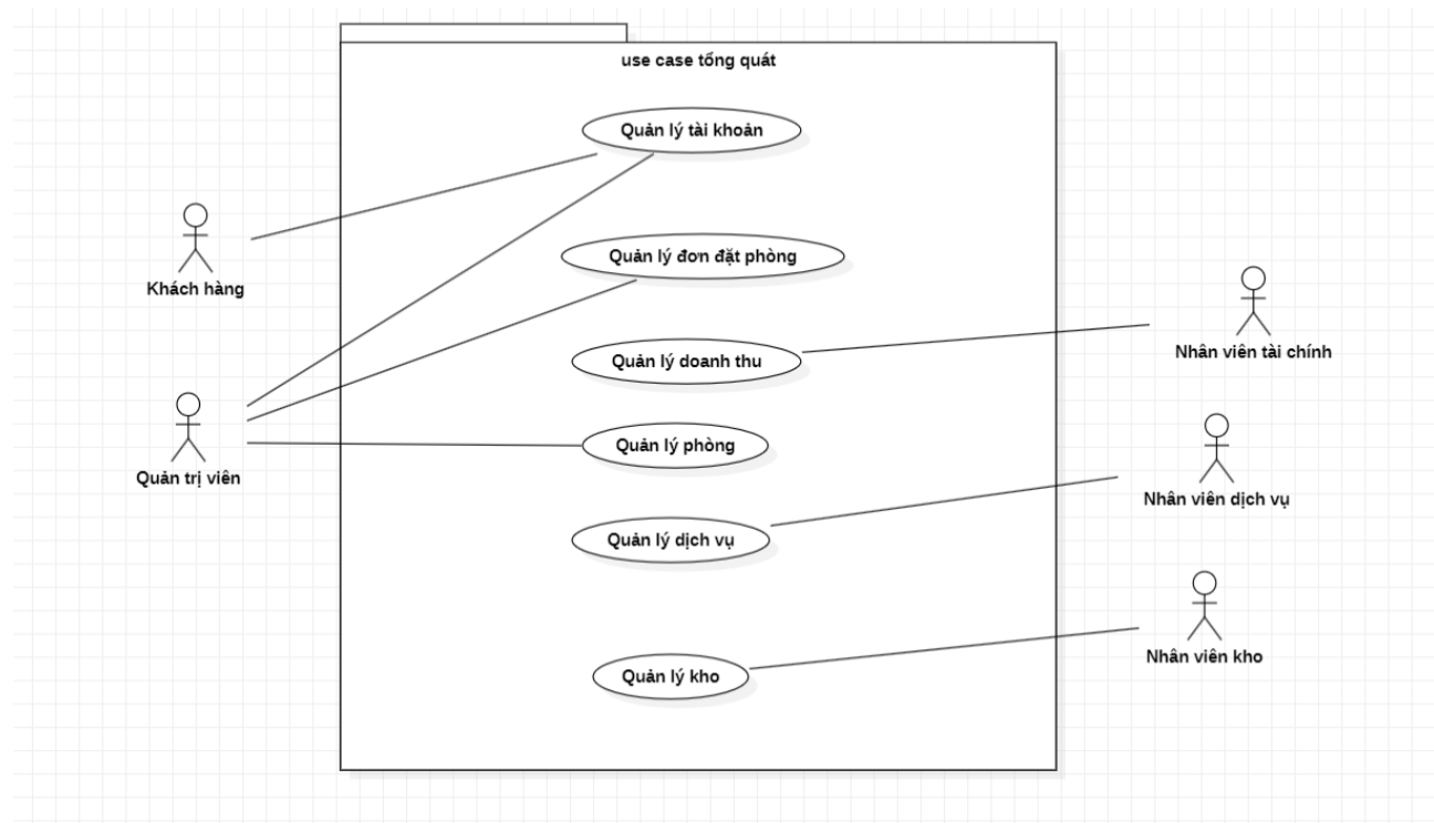
Use case tổng quát
