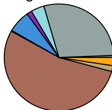
t\bar{t} + \text{light} CR
