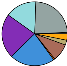
t\bar{t} + 1B CR
