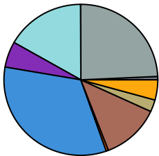
t\bar{t} + 1b CR
