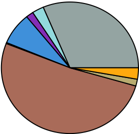
t\bar{t} + \text{light} CR
