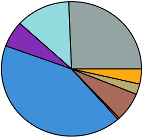
t\bar{t} + 1b CR
