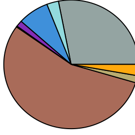
t\bar{t} + \text{light} region
