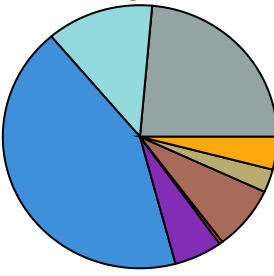
t\bar{t} + 1b region
