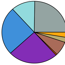
t\bar{t} + B region
