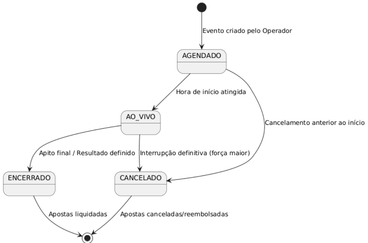
[DIAGRAMA DE ESTADOS - EVENTO]
