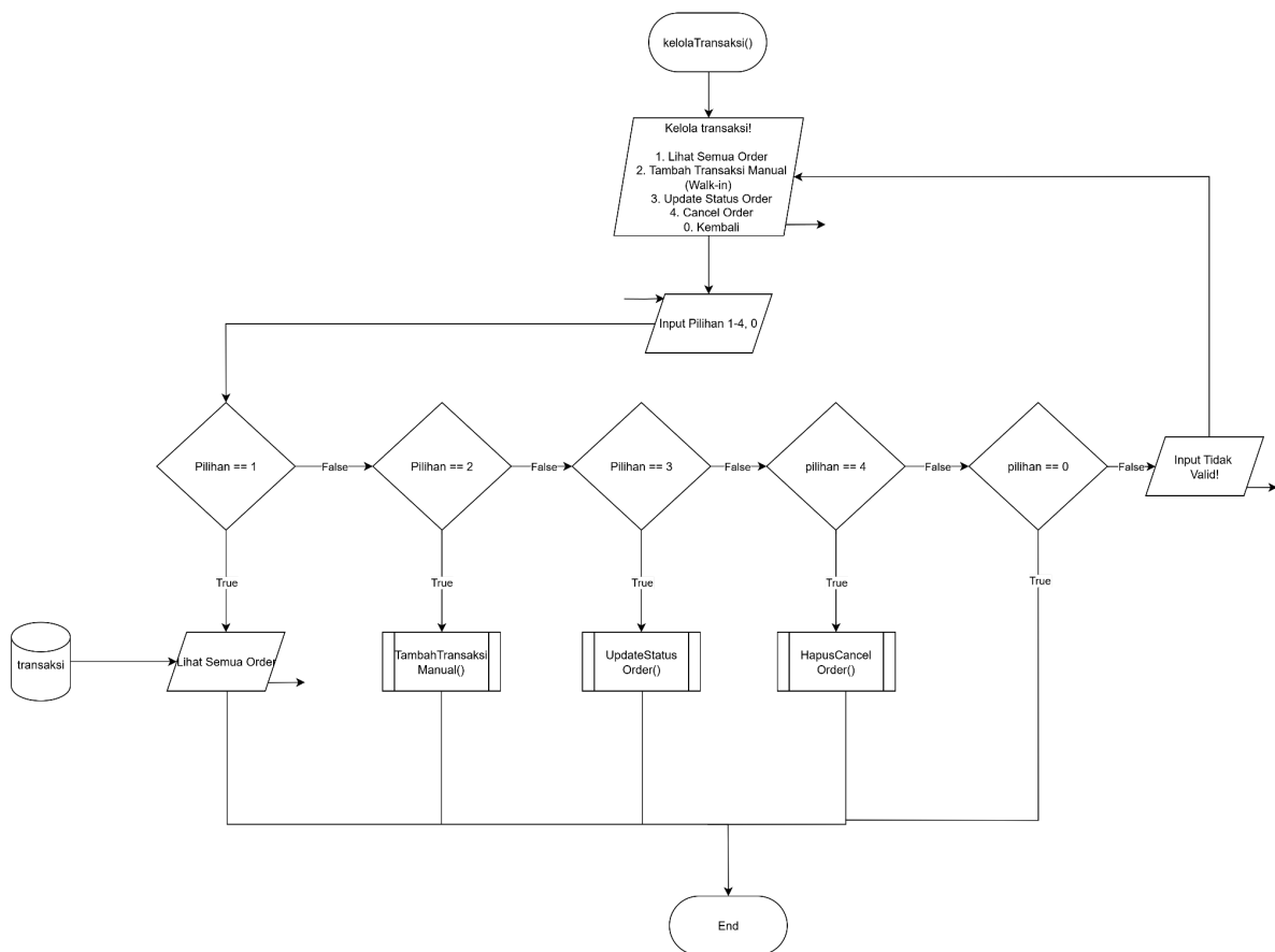
Gambar 2.11 Flowchart Fungsi Kelola Transaksi
