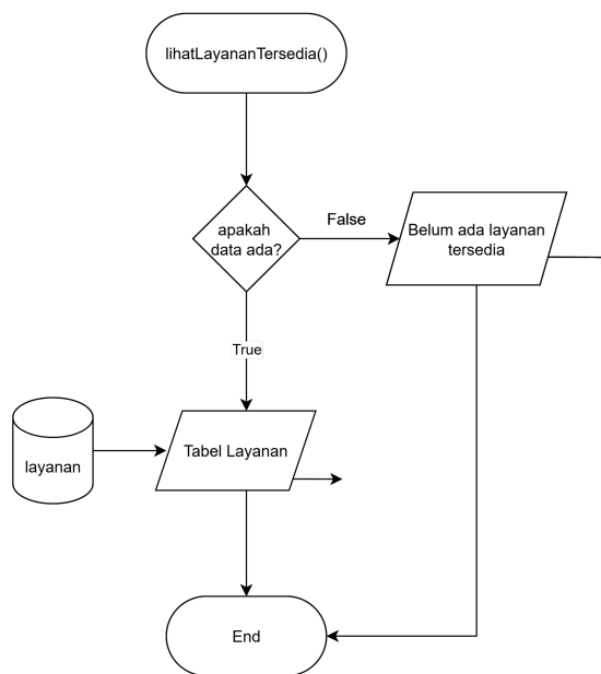
Gambar 2.7 Flowchart Fungsi Lihat Layanan Tersedia
