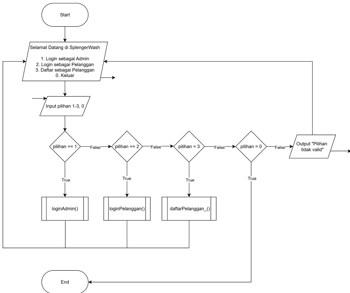
Gambar 2.1 Flowchart Menu Utama
