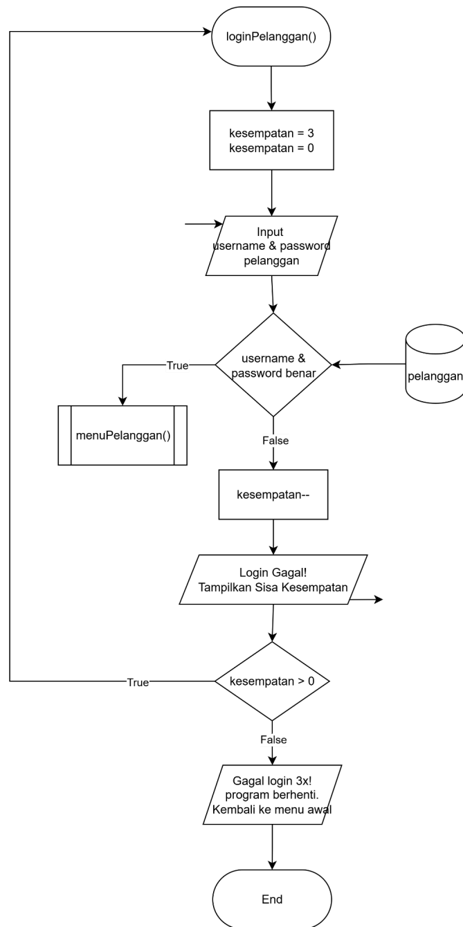
Gambar 2.3 Flowchart Fungsi Login Pelanggan
