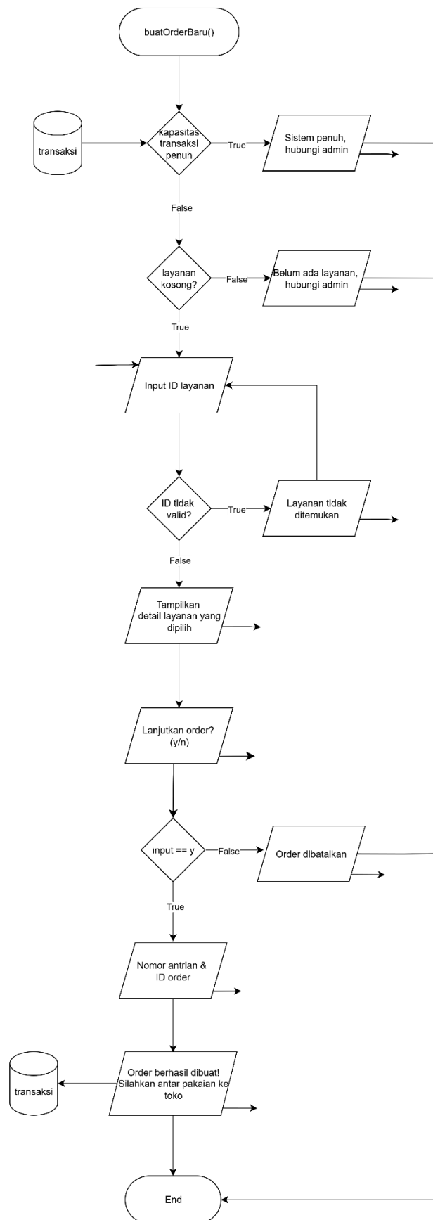
Gambar 2.19 Flowchart Fungsi Buat Order Baru
