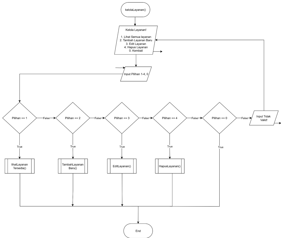
Gambar 2.6 Flowchart Fungsi Kelola Layanan
