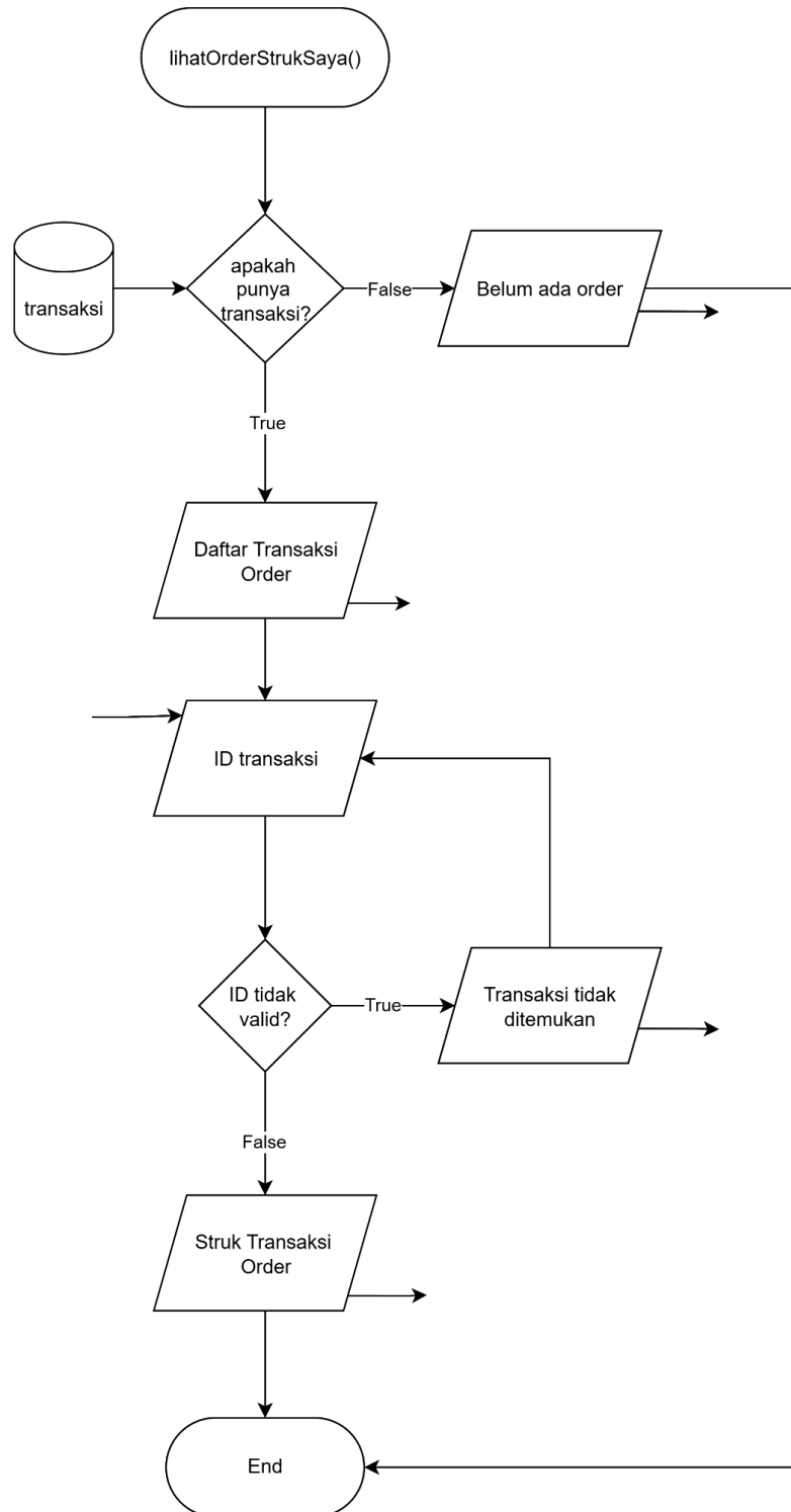
Gambar 2.20 Flowchart Fungsi Lihat Order Struk Saya
