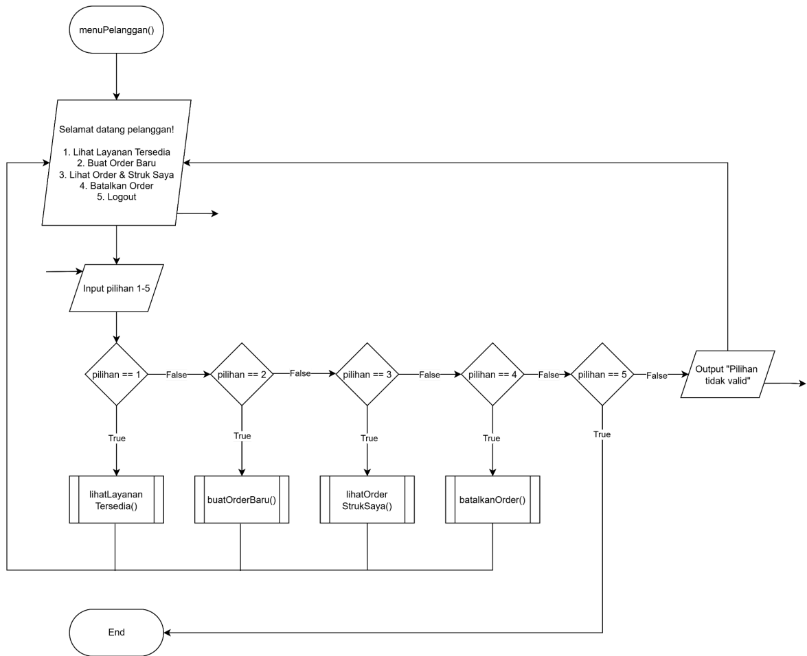
Gambar 2.18 Flowchart Fungsi Menu Pelanggan
