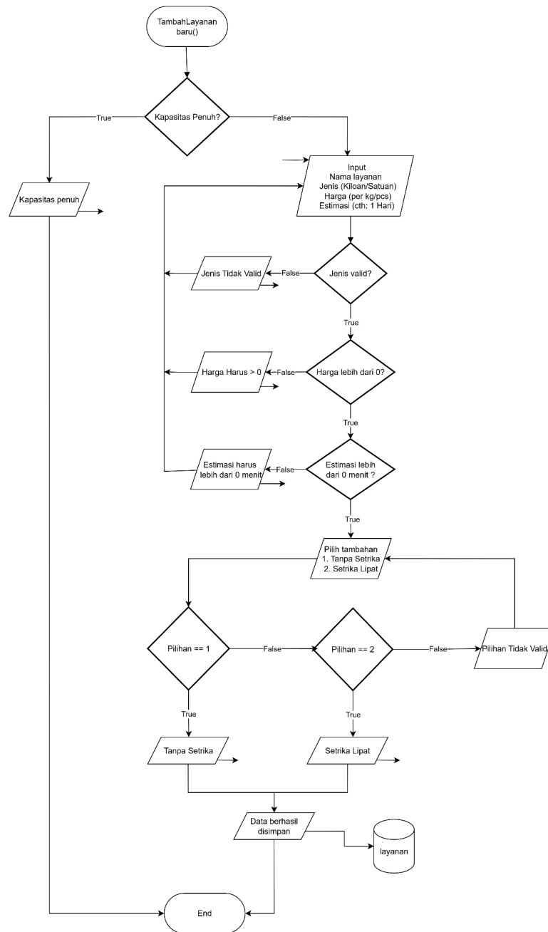
Gambar 2.8 Flowchart Fungsi Tambah Layanan Baru
