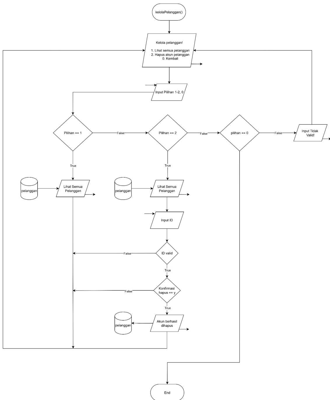
Gambar 2.17 Flowchart Fungsi Kelola Pelanggan
