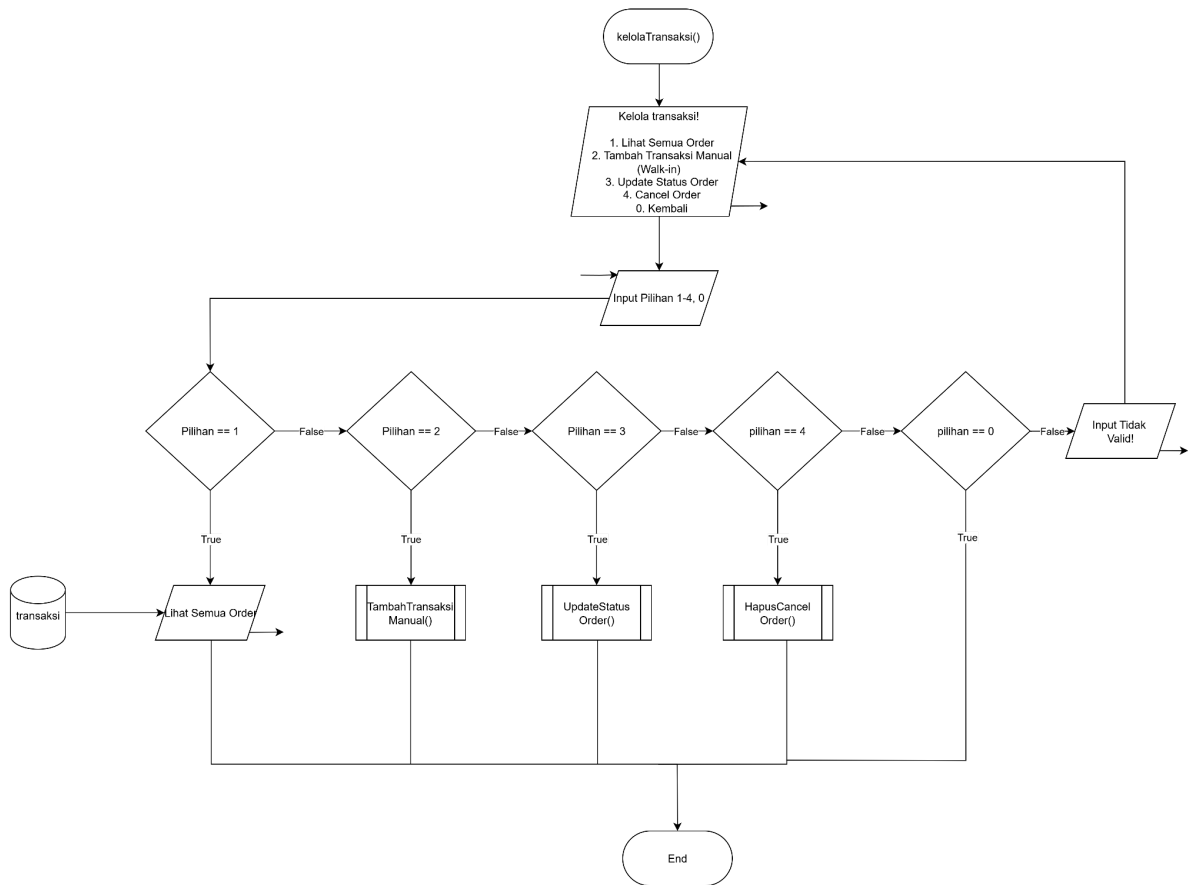
Gambar 2.11 Flowchart Fungsi Kelola Transaksi
