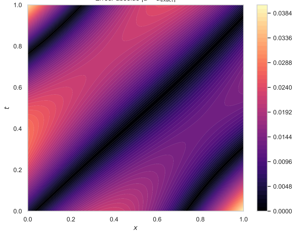
Erreur absolue |\hat{u} - u_{\text{exact}}|
