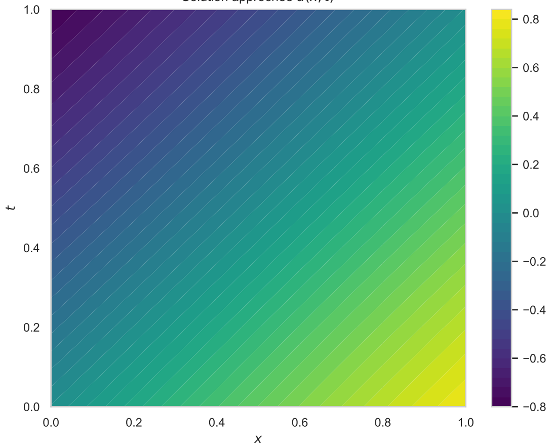
Solution approchée \hat{u}(x, t)
