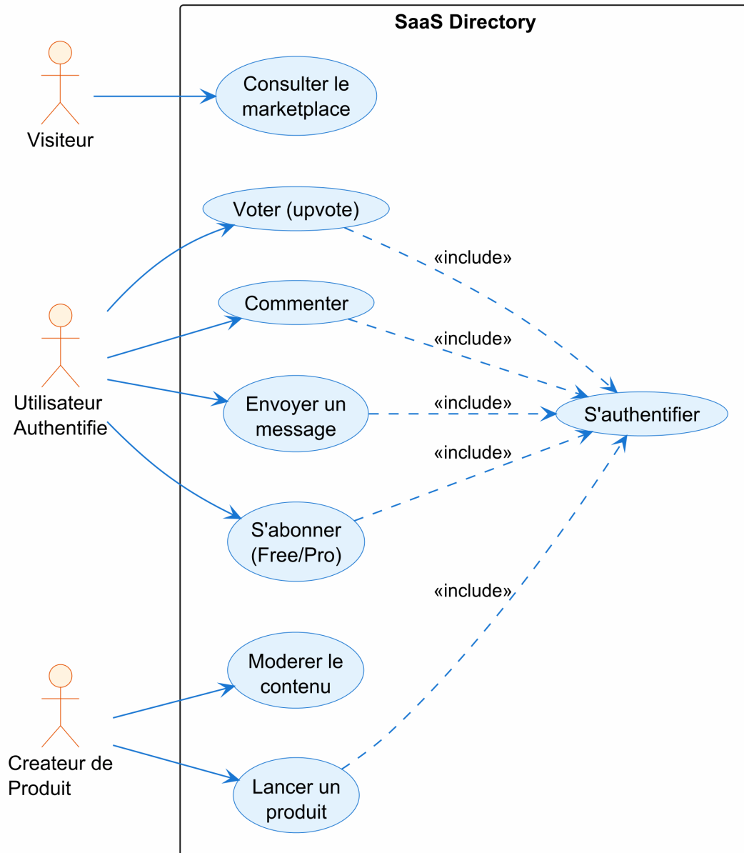
Diagramme de Cas d'Utilisation --- SaaS Directory
