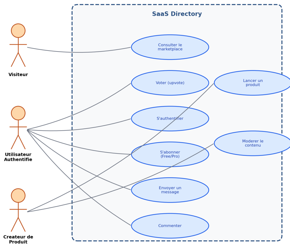
FIGURE 4 – Diagramme de Cas d'Utilisation — SaaS Directory
