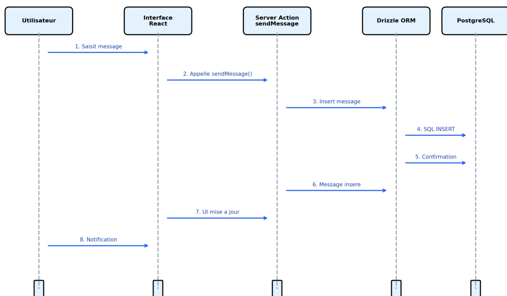
Diagramme de Sequence --- Envoi d'un Message
