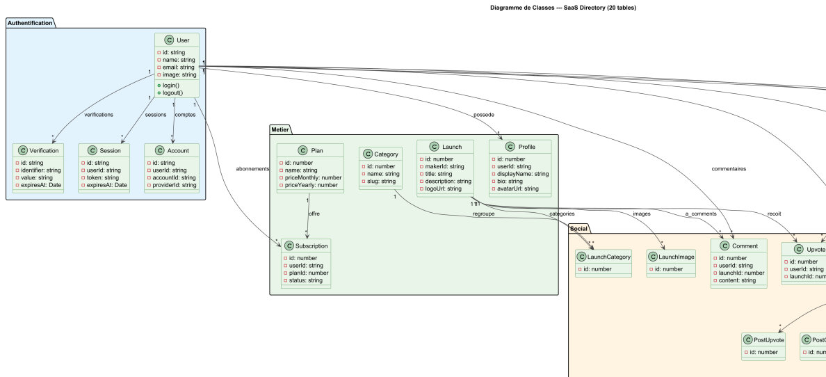
FIGURE 5 – Diagramme de Classes (20 tables)
