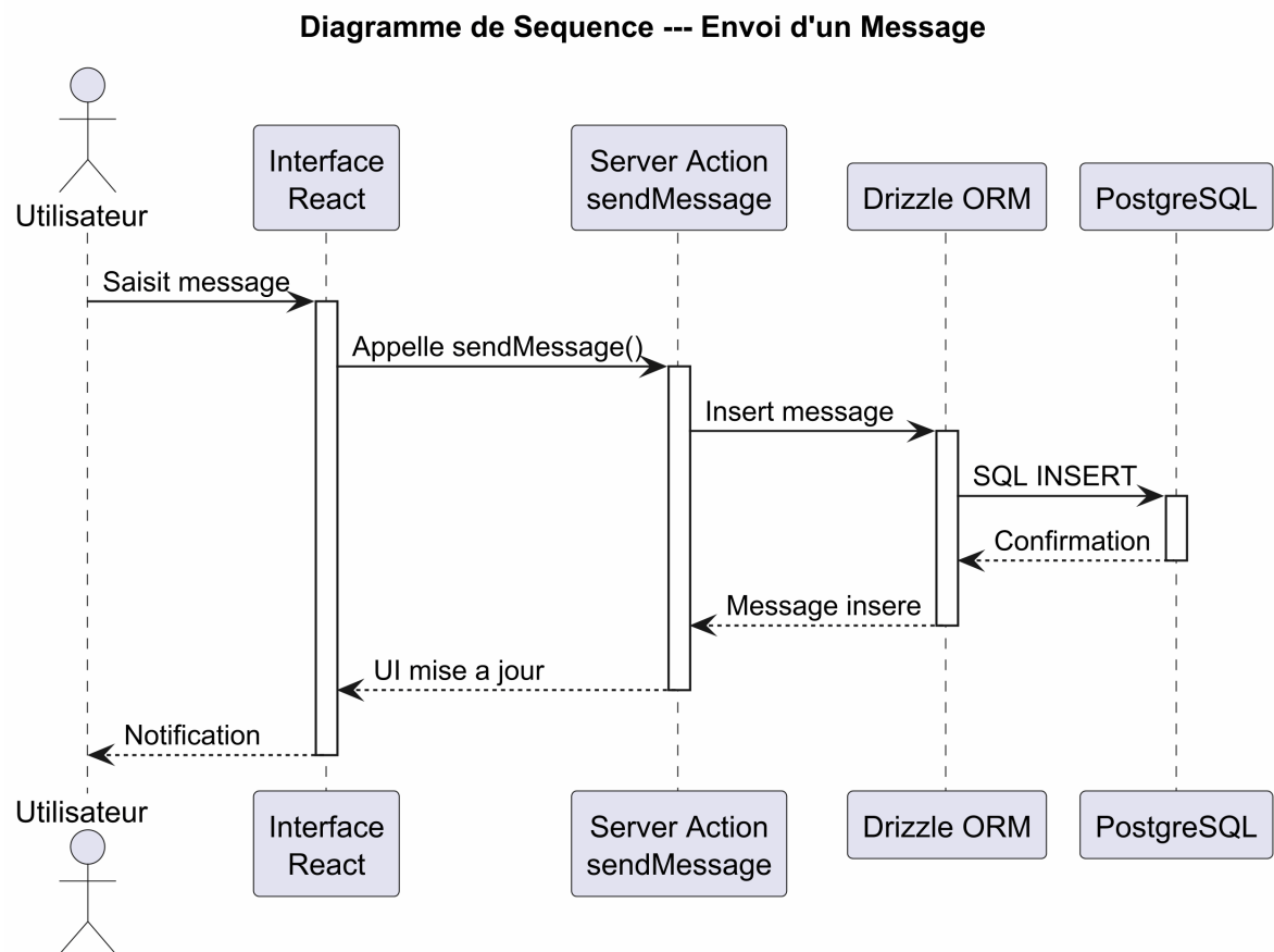
FIGURE 6 – Diagramme de Séquence — Envoi d'un Message
