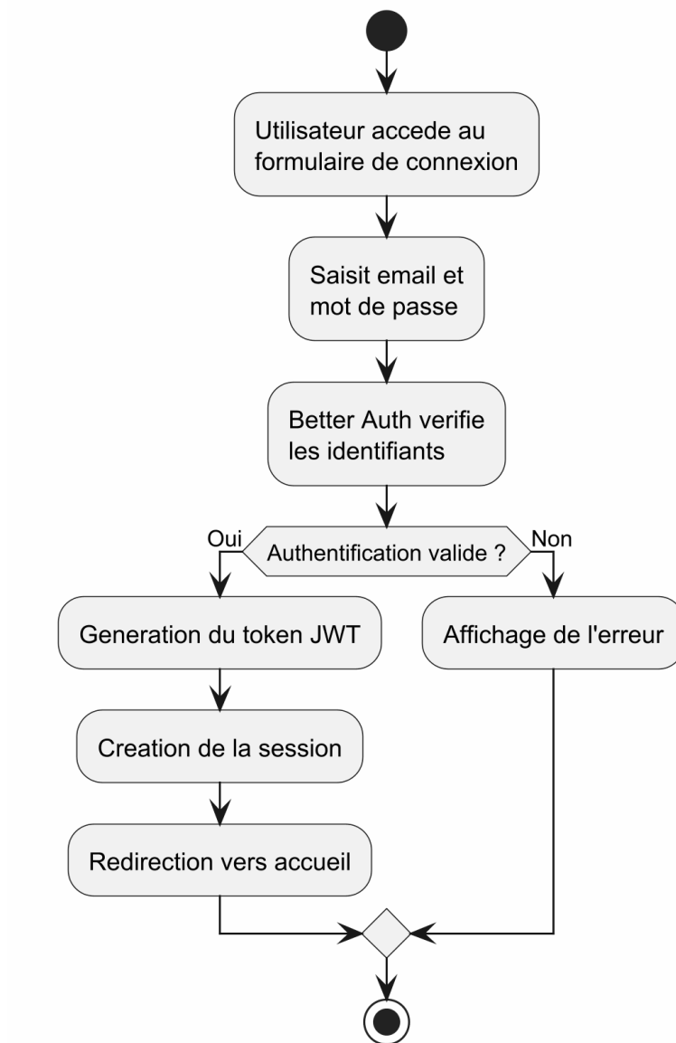
FIGURE 2 – Diagramme d'Activité — Flux d'Authentification
