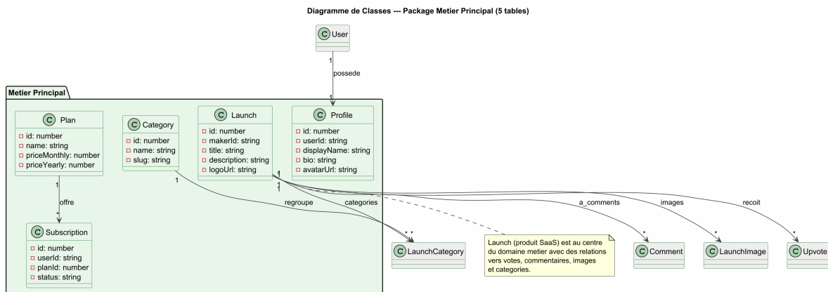
FIGURE 6 – Diagramme de Classes — Package Métier Principal (5 tables)
