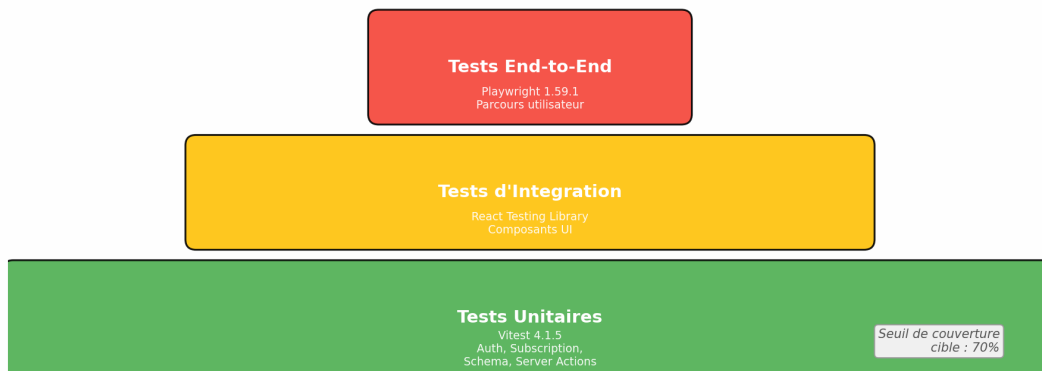
FIGURE 9 – Pyramide des Tests — Stratégie de validation de SaaS Directory
