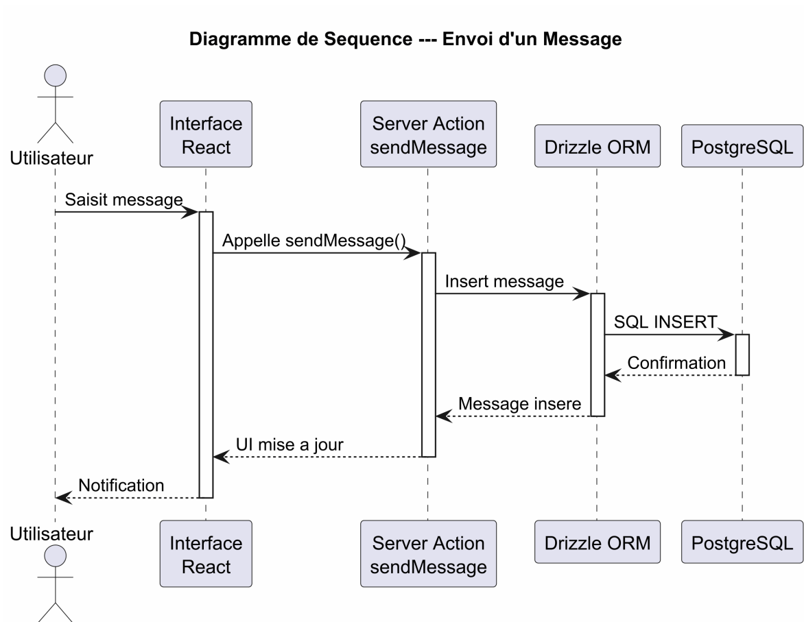
FIGURE 8 – Diagramme de Séquence — Envoi d'un Message
