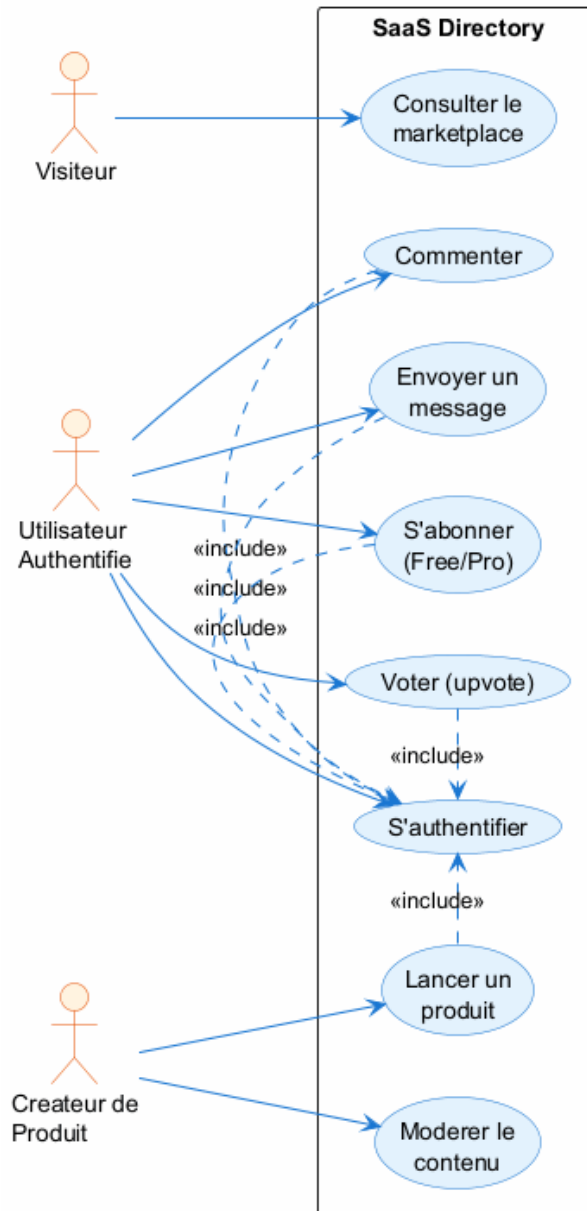
Diagramme de Cas d'Utilisation --- SaaS Directory
