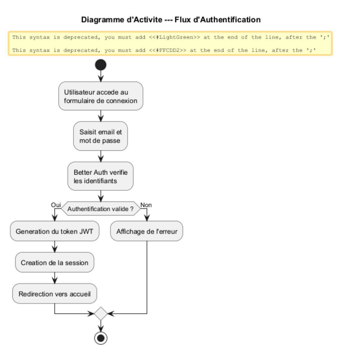
FIGURE 2 – Diagramme d'Activité — Flux d'Authentification
