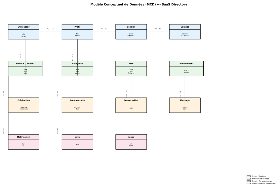
FIGURE 4 – Modèle Conceptuel de Données (MCD) — SaaS Directory
