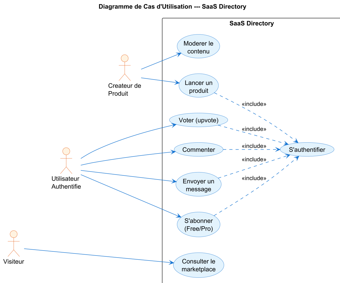
FIGURE 6 – Diagramme de Cas d'Utilisation — SaaS Directory
