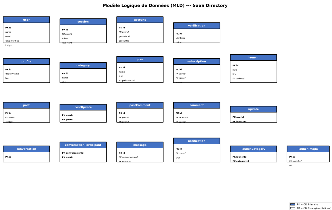
FIGURE 5 – Modèle Logique de Données (MLD) — SaaS Directory
