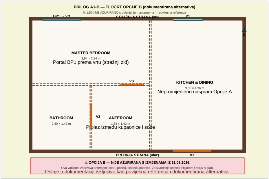
M 1:50 | NE AŽURIRANO s izmjenama R8 — povijesna referenca
